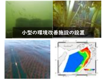
刀養殖の状況 (地独)大阪府立環境農林水産総合研究所 夏季底層DO分布図 (2019～2021年度8月平均)
