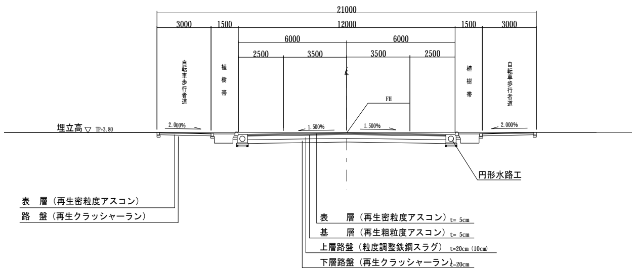
汐見沖1号線 (21m道路 標準部)
