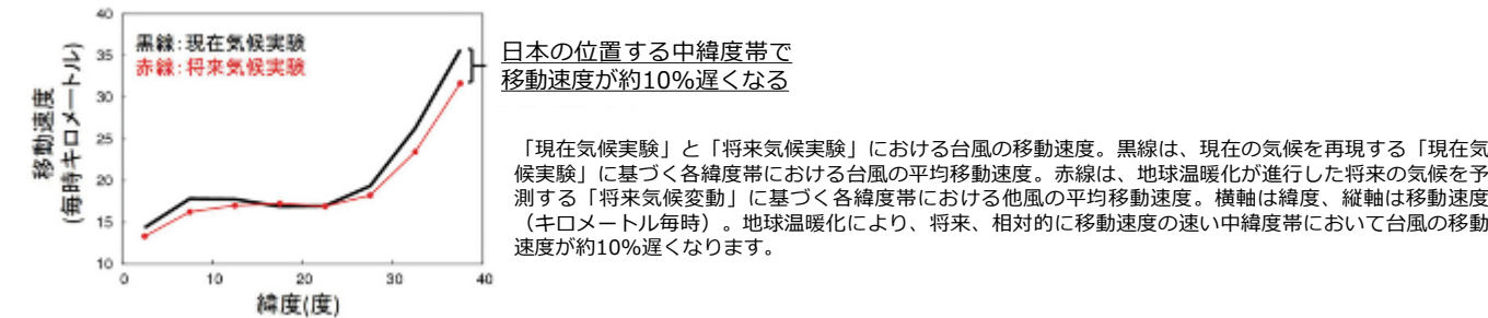
緯度別の台風の移動速度の変化
