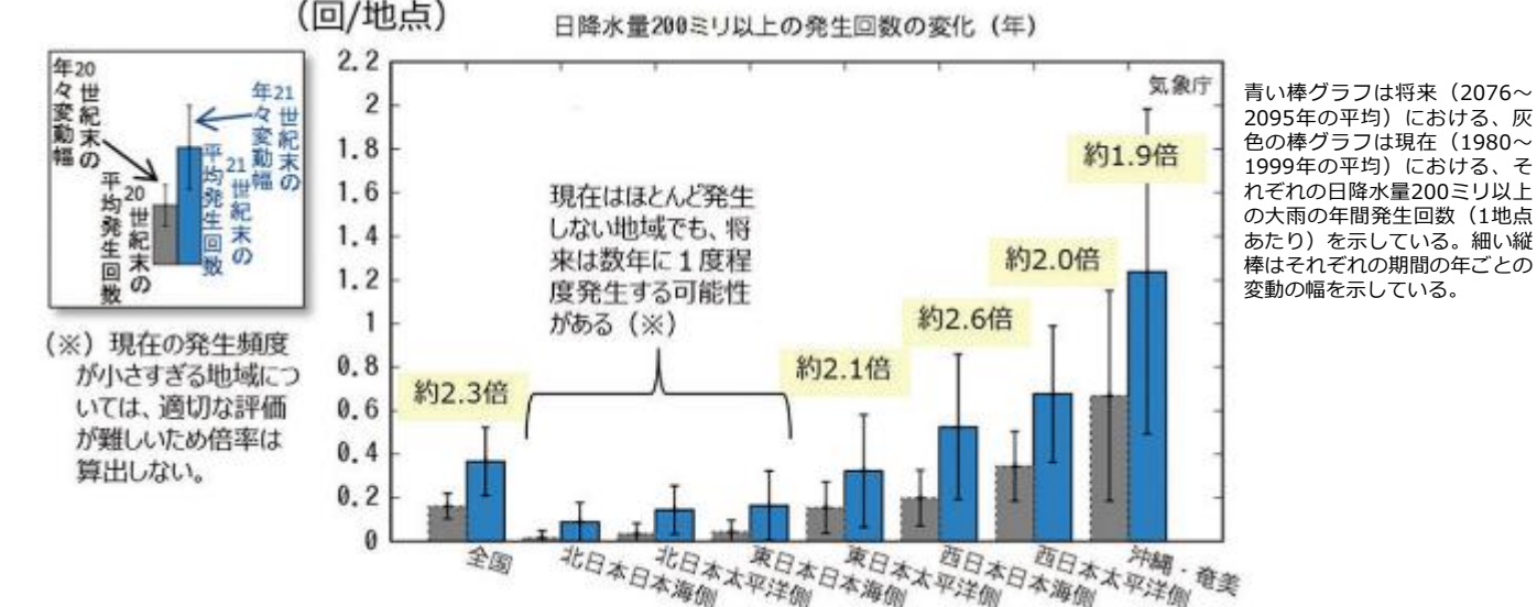
日降水量200ミリ以上の大雨の年間発生回数の変化(二酸化炭素の排出が高いレベルで続く場合)
