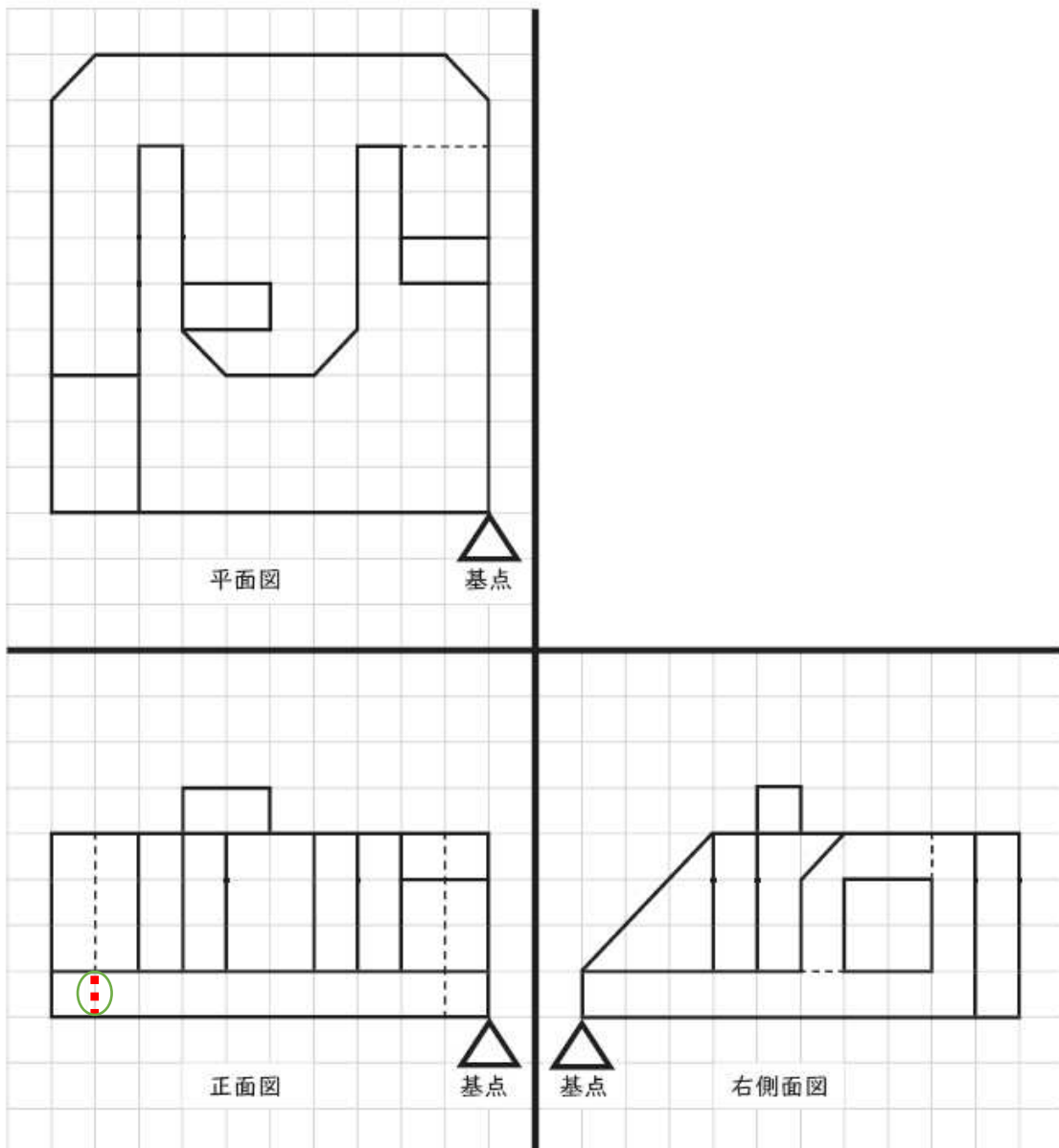
図 正投影図(三面図)
