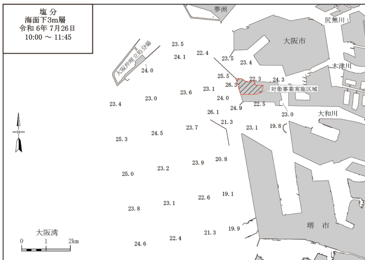
第 10.1.2.1-5 図(3) 塩分水平分布 (夏季)
