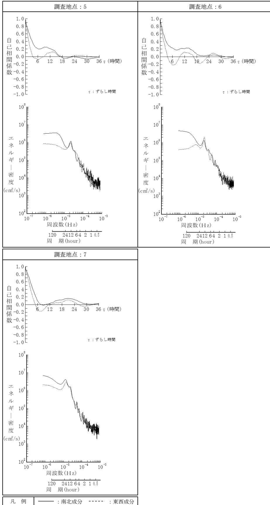
第 10.1.2.1-11 図(4) 流速変動の自己相関係数とエネルギースペクトラム（夏季）
