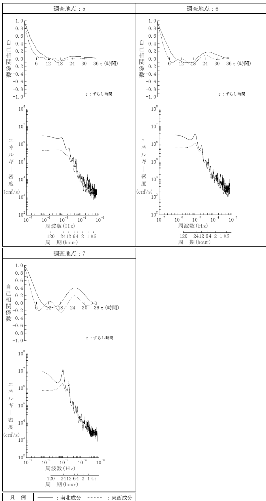
第 10. 1. 2. 1-11 図(8) 流速変動の自己相関係数とエネルギースペクトラム (冬季)
