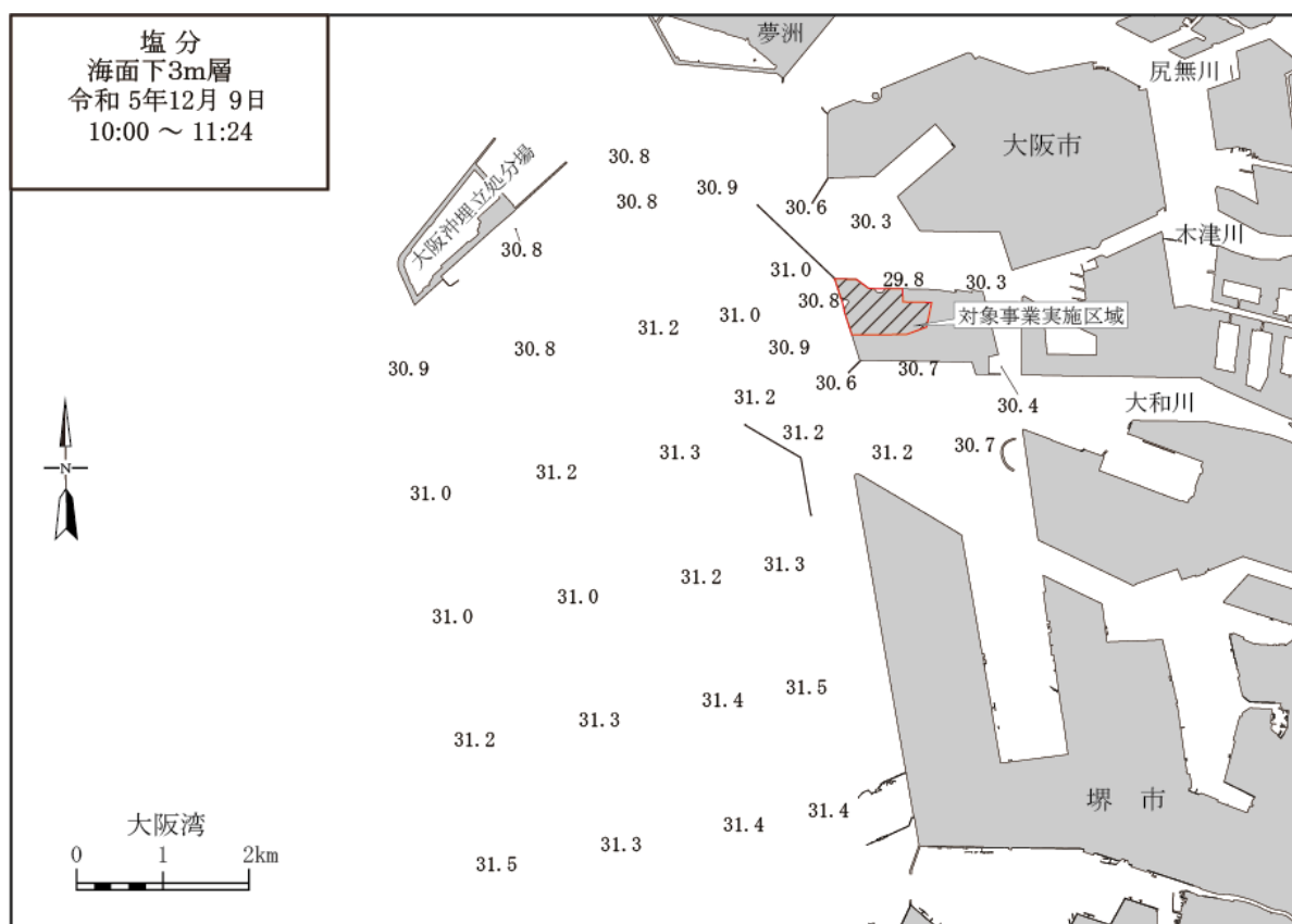
第 10.1.2.1-5 図(5) 塩分水平分布 (秋季)
