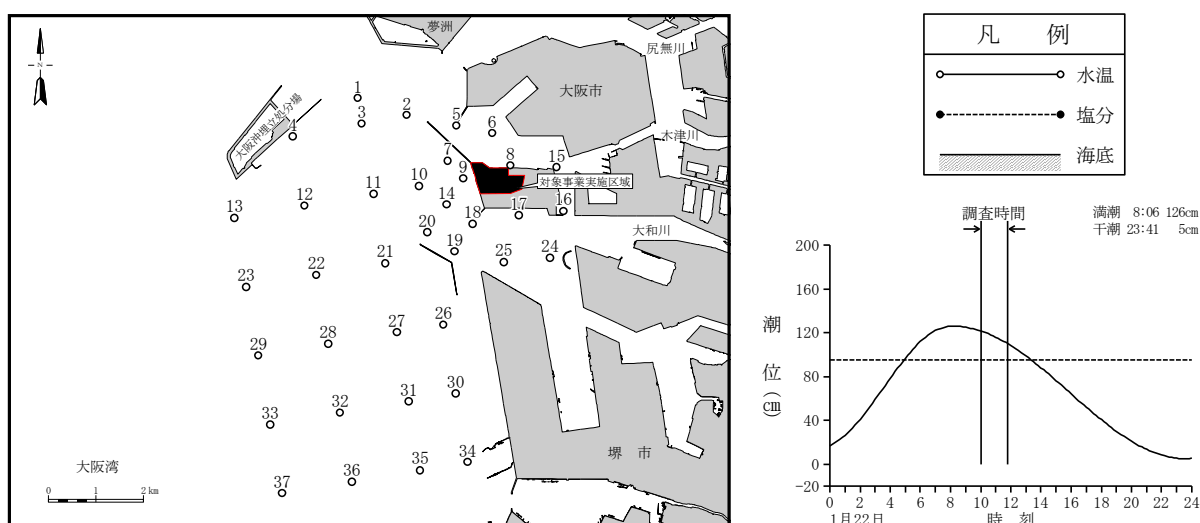
第 10. 1. 2. 1-6 図(10) 水温・塩分の鉛直分布 (冬季)
