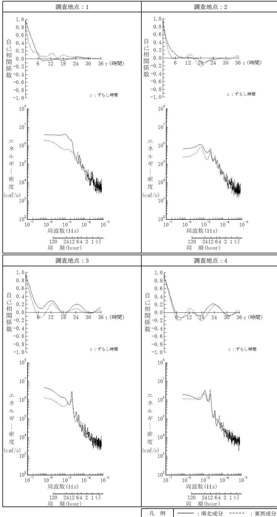
第 10. 1. 2. 1-11 図(1) 流速変動の自己相関係数とエネルギースペクトラム（春季）
