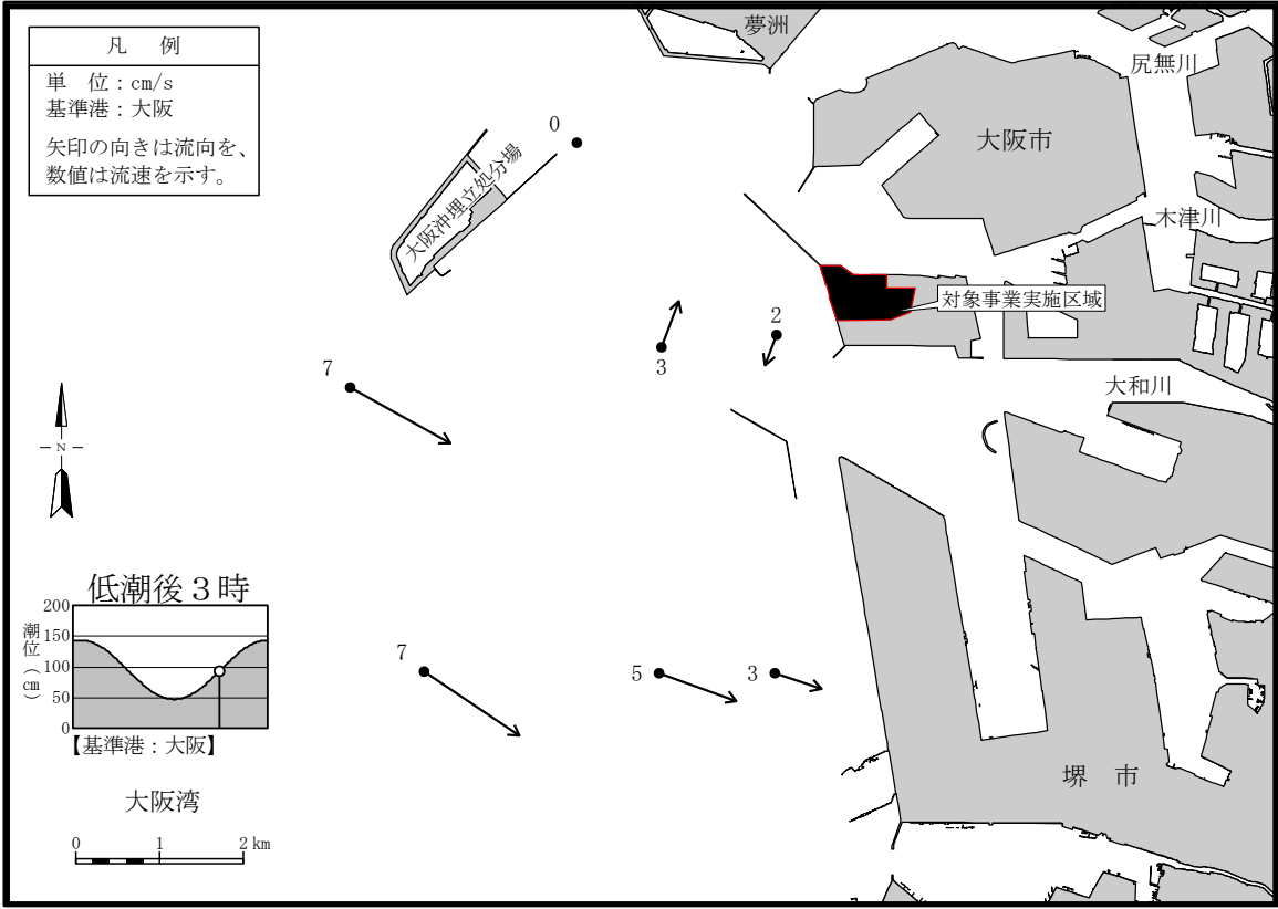
第 10. 1. 2. 1-10 図(6) 平均大潮期の流況（秋季）
