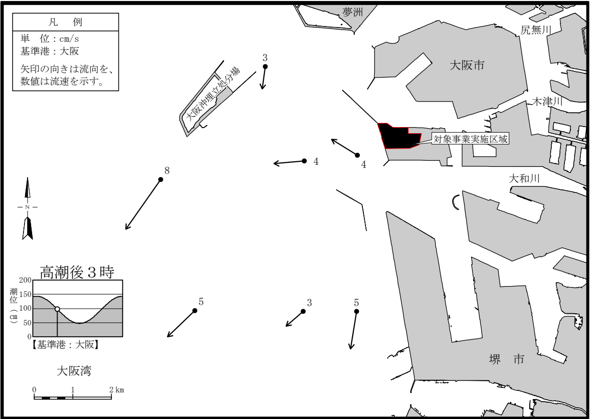
第 10. 1. 2. 1-10 図(5) 平均大潮期の流況（秋季）
