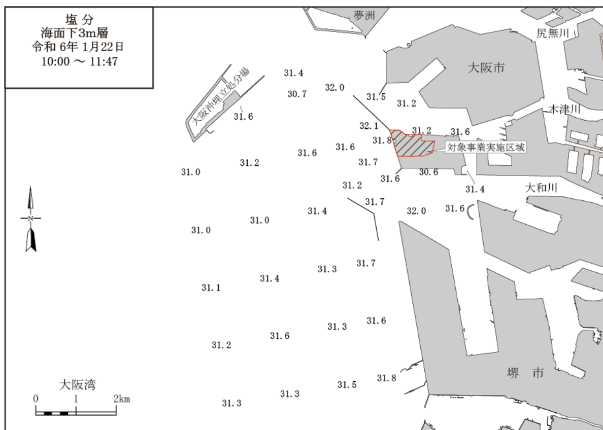
第 10.1.2.1-5 図(7) 塩分水平分布 (冬季)
