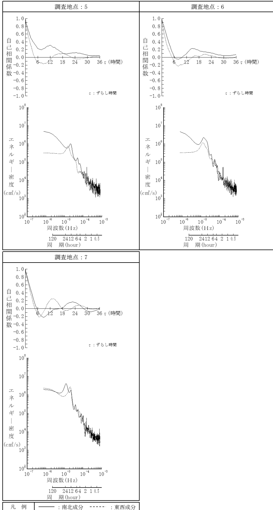
第 10. 1. 2. 1-11 図(2) 流速変動の自己相関係数とエネルギースペクトラム (春季)
