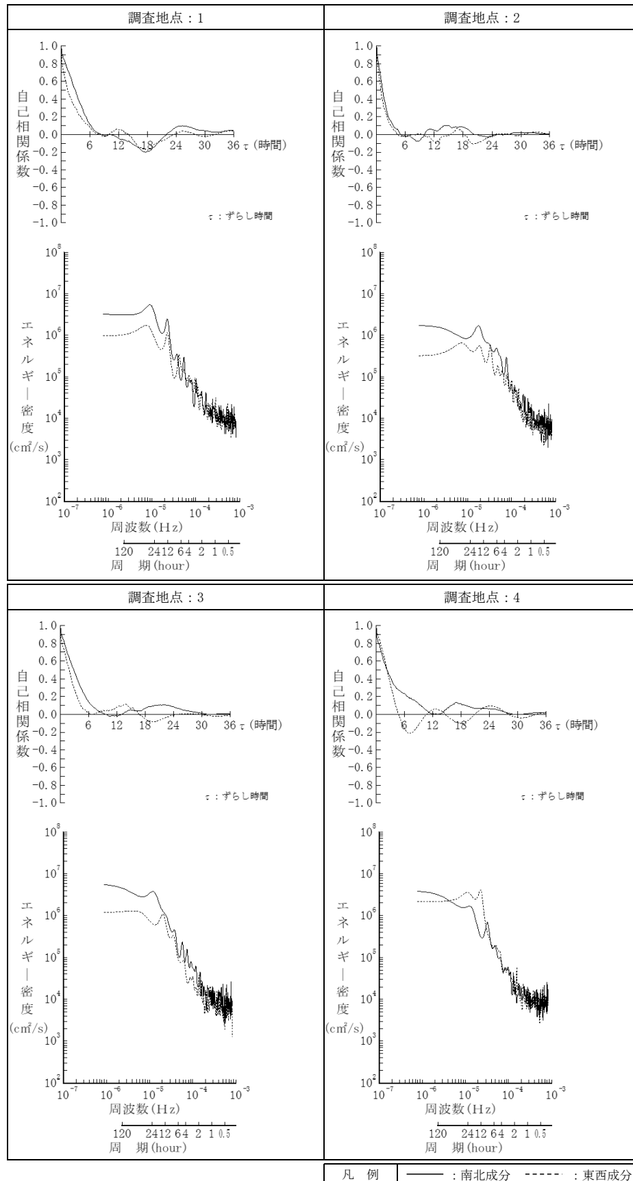
第 10.1.2.1-11 図(3) 流速変動の自己相関係数とエネルギー Spektrum (夏季)
