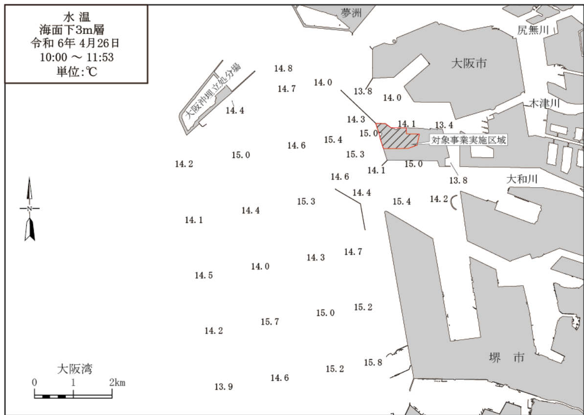
第 10.1.2.1-4 図(1) 水温水平分布 (春季)
