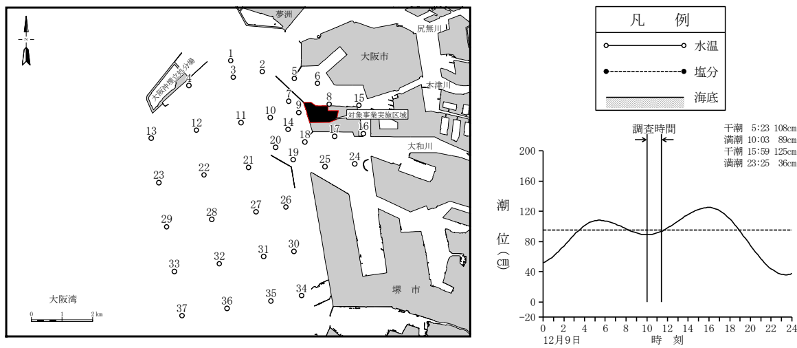
第 10. 1. 2. 1-6 図(7) 水温・塩分の鉛直分布（秋季）
