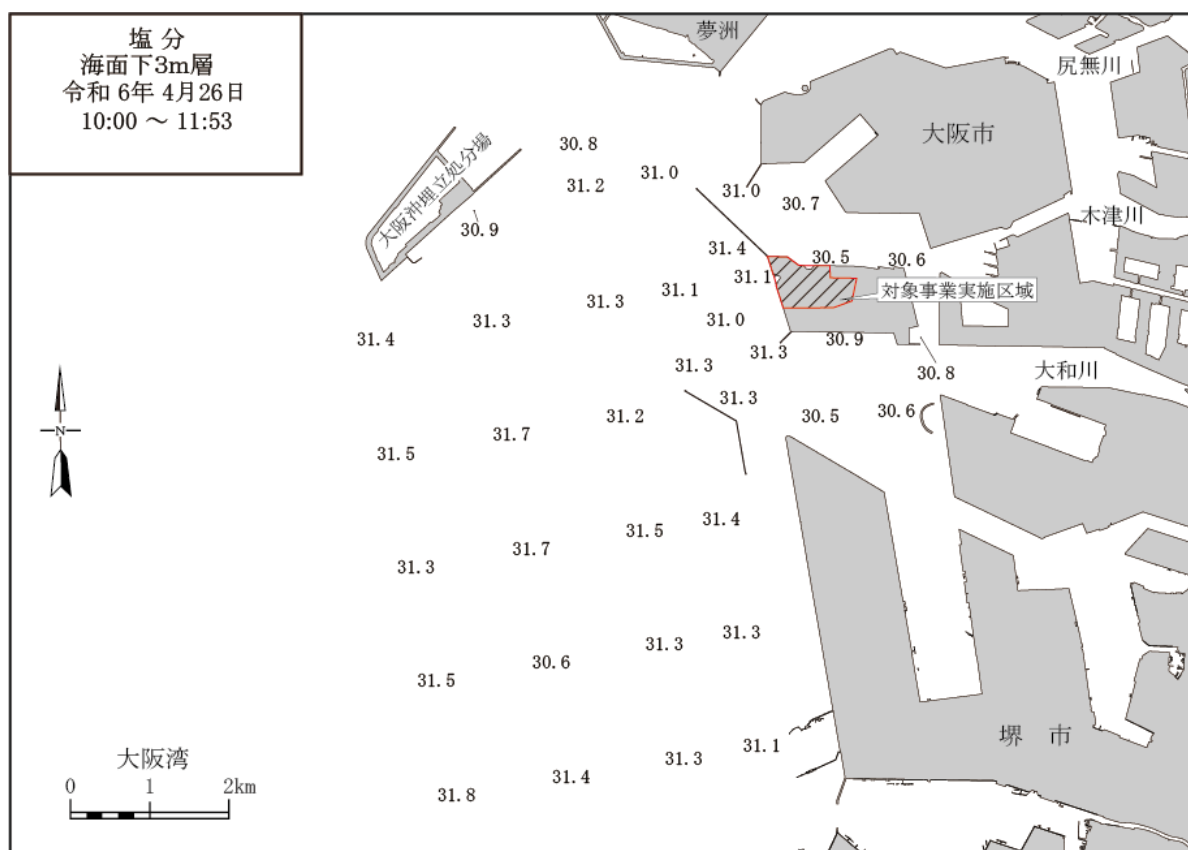
第 10.1.2.1-5 図(1) 塩分水平分布 (春季)
