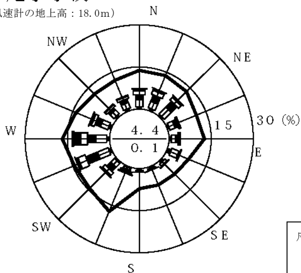
第 4.3.1-2 図 平尾小学校局における年間風配図及び平均風速（令和 3 年度）
