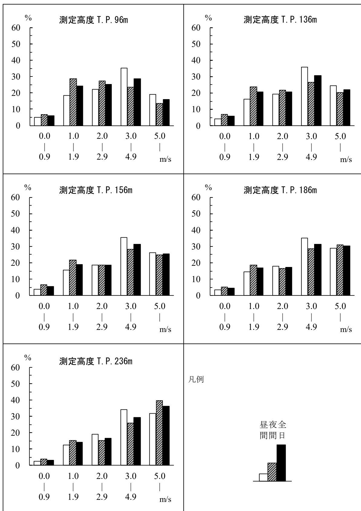
図 7. 1－10（1） 風速階級別出現頻度（測定高度：T. P. 96m～236m、全日）
