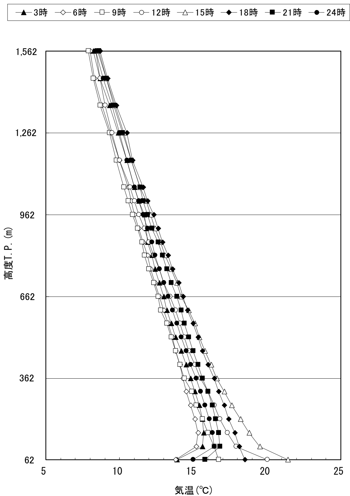
図7. 1-12 (1) 平均気温及び気温勾配の鉛直分布 (年間)
