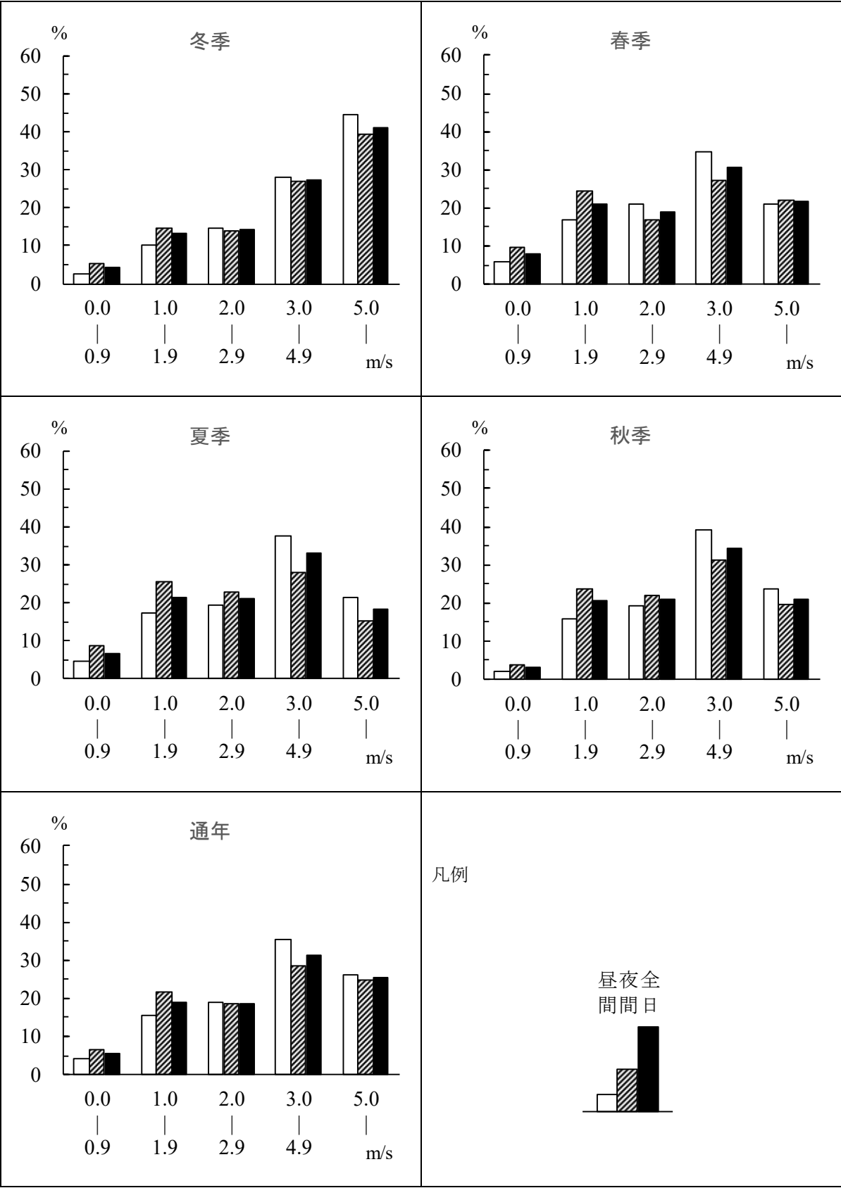
图 7. 1-8 风速階級別出現頻度 (上層風)
