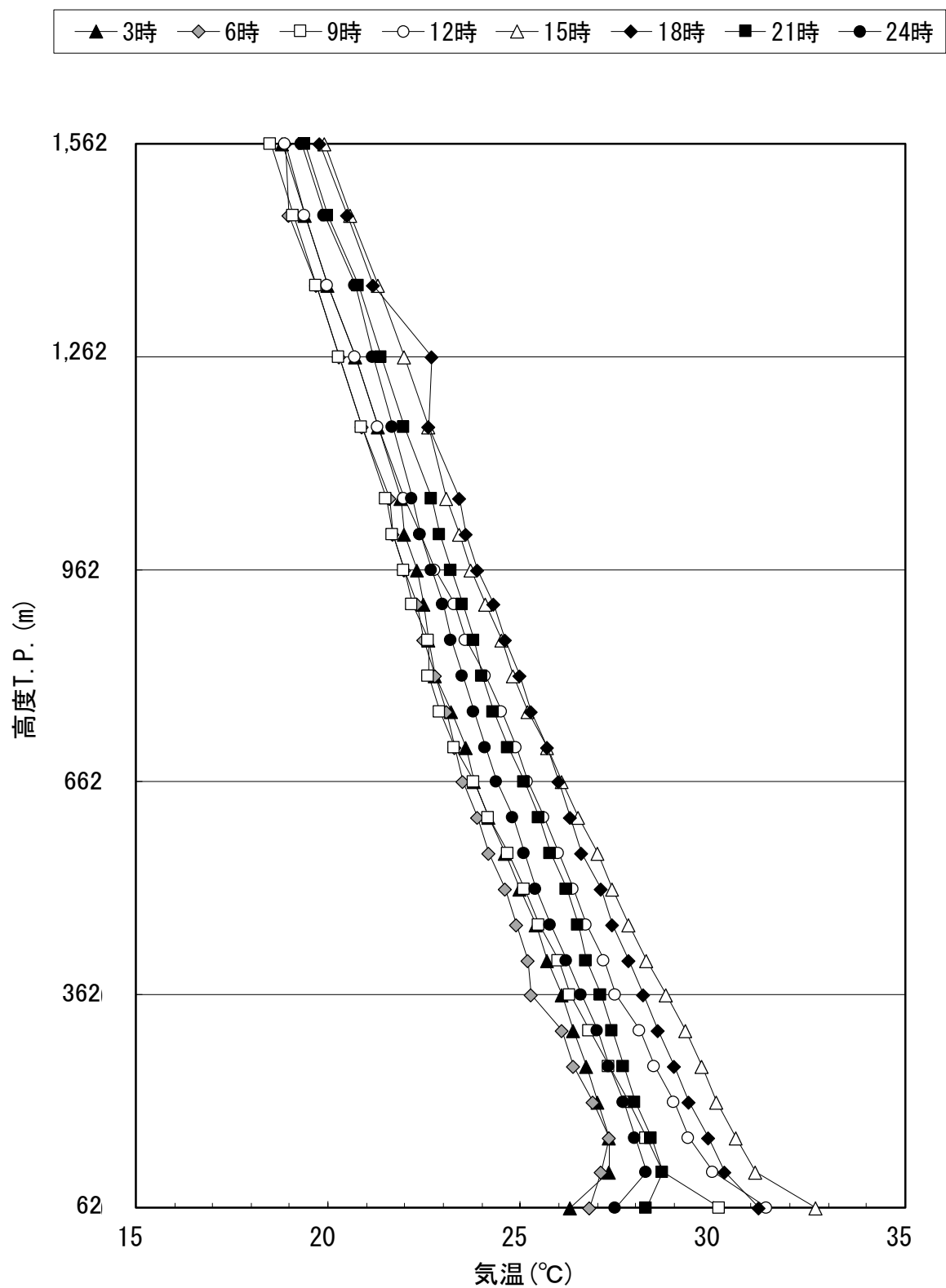
図7. 1-12(4) 平均気温及び気温勾配の鉛直分布 (夏季)
