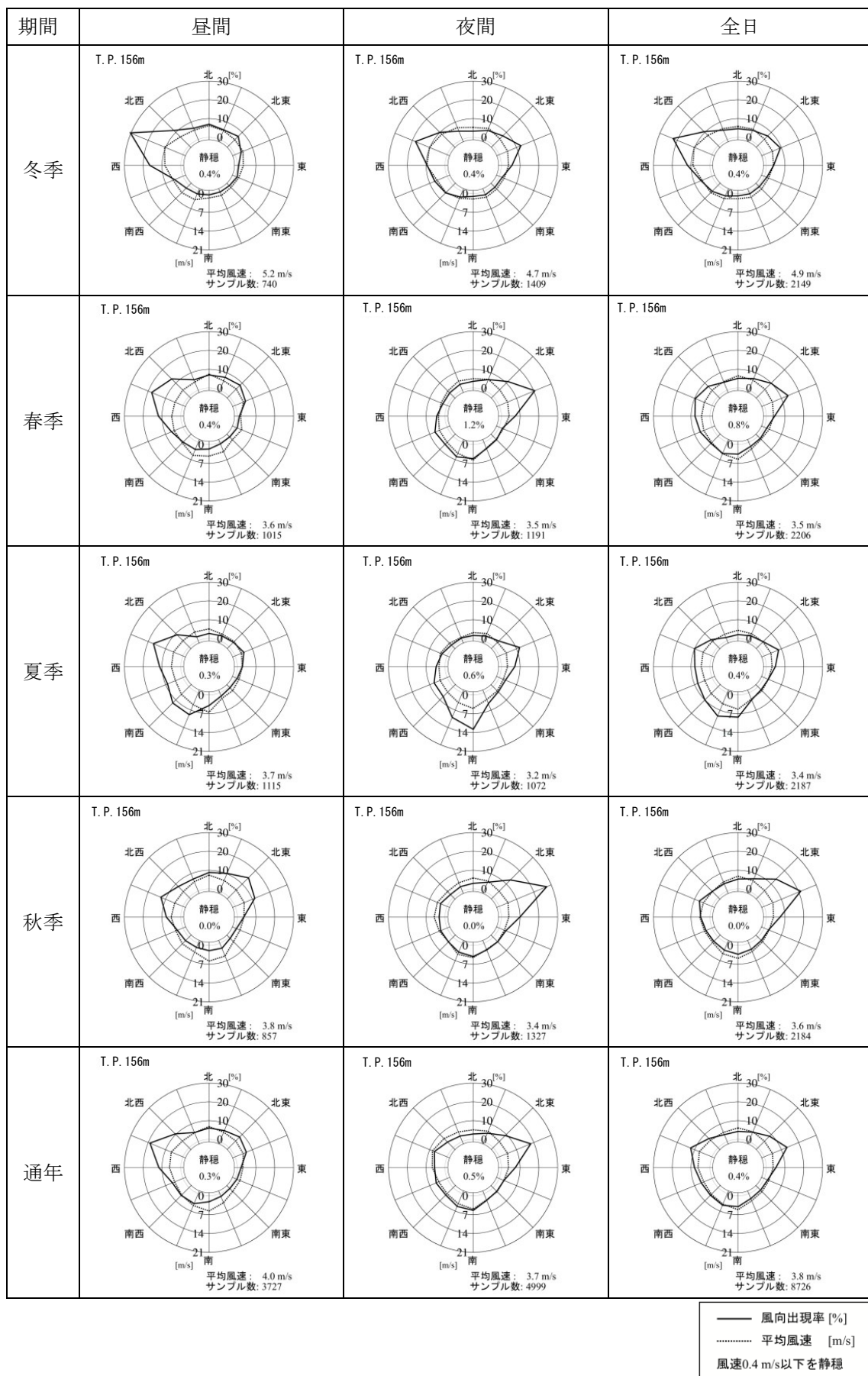
図 7. 1-7 風配図及び風向別平均風速（上層風）
