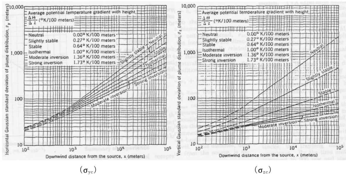
図 7. 1 - 2 1 カーペンターらの煙の拡がり幅
