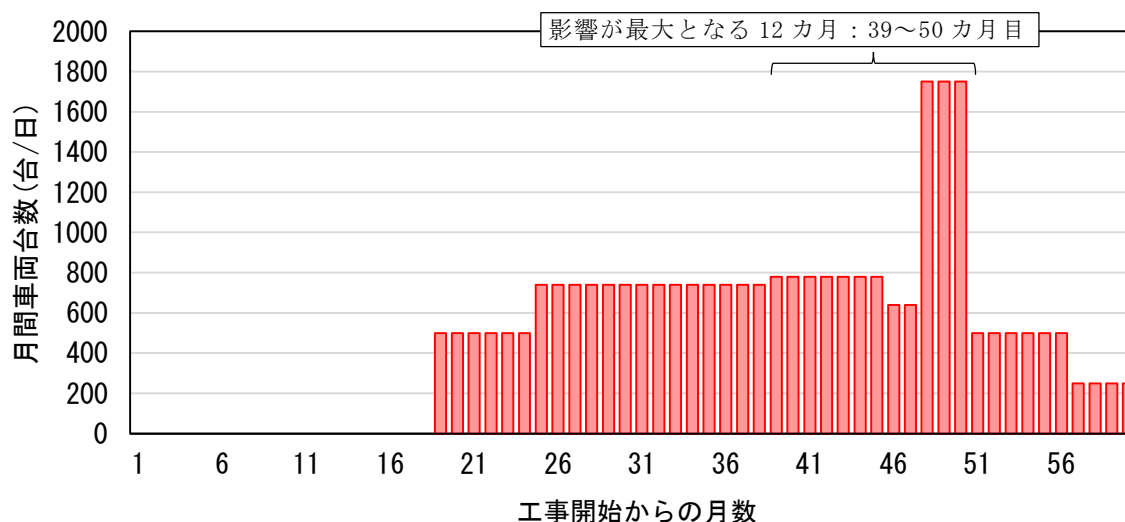
図7. 1-45 大型車の年間交通量の時系列変化
