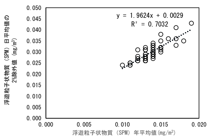
図 7. 1 - 2 6 浮遊粒子状物質濃度の年平均値と日平均値の年間 2%除外値の関係
