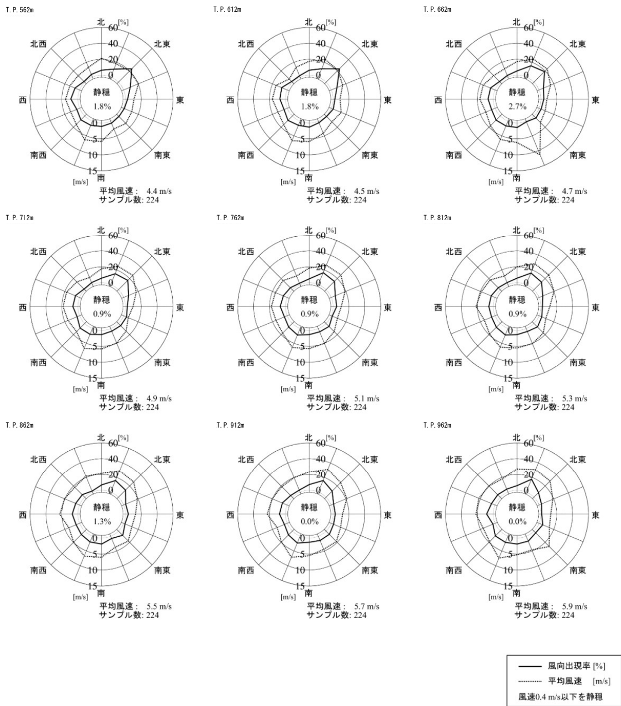
図7. 1－11（2） 高度別風配図及び風向別平均風速（測定高度：T. P. 562m～962m）
