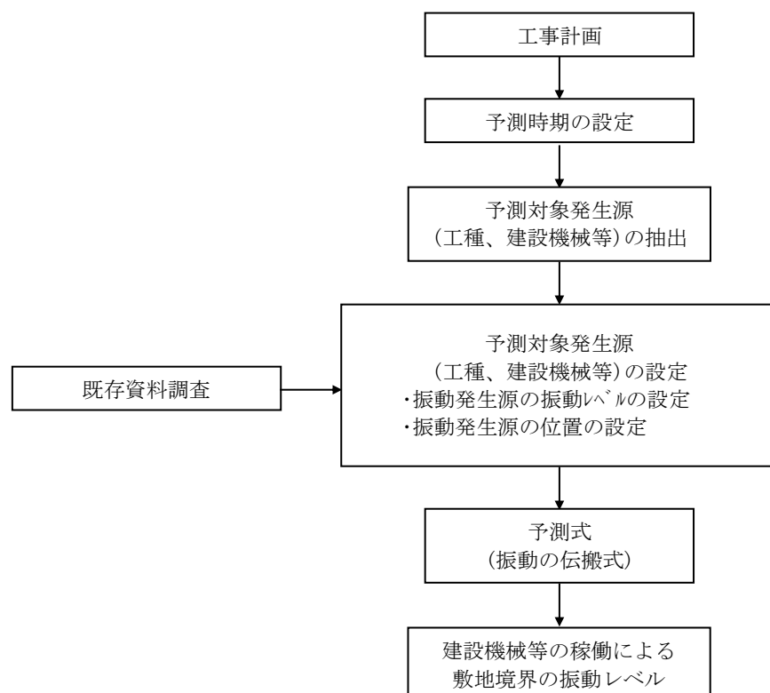
図 7-3-8 施設の建設に伴う振動の予測手順
