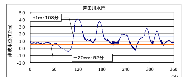
芦田川水門の水位変化
