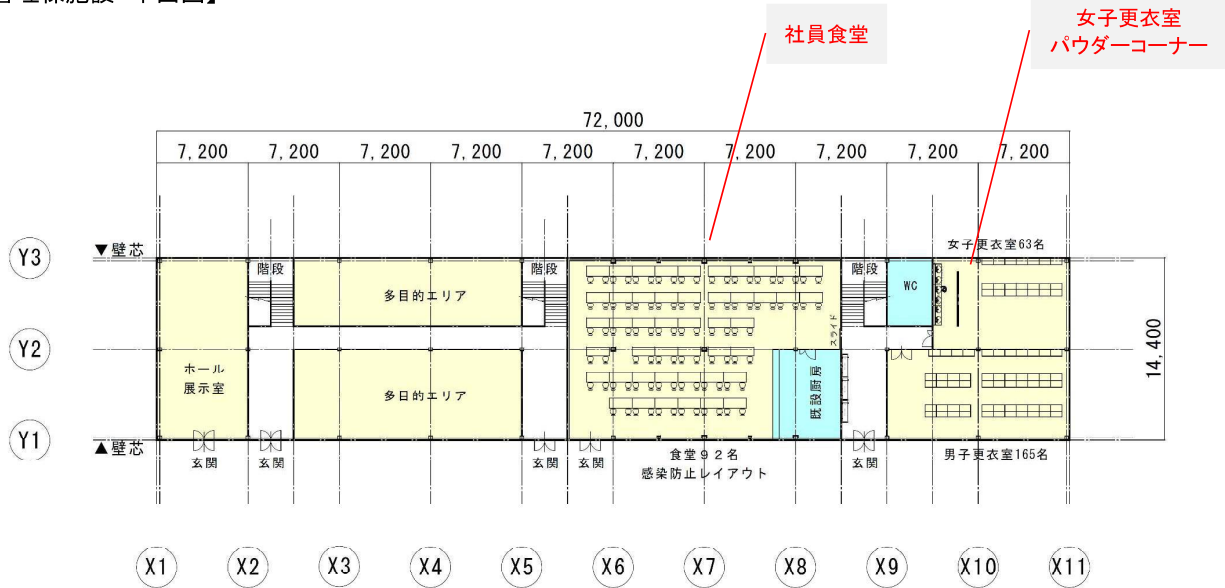
1階平面図
