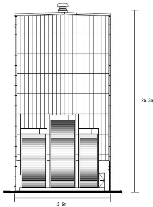
(西側立面図)
