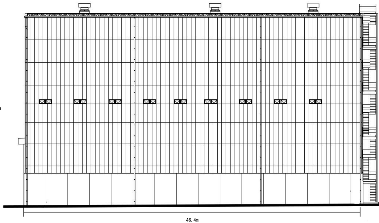
(南側立面図)
