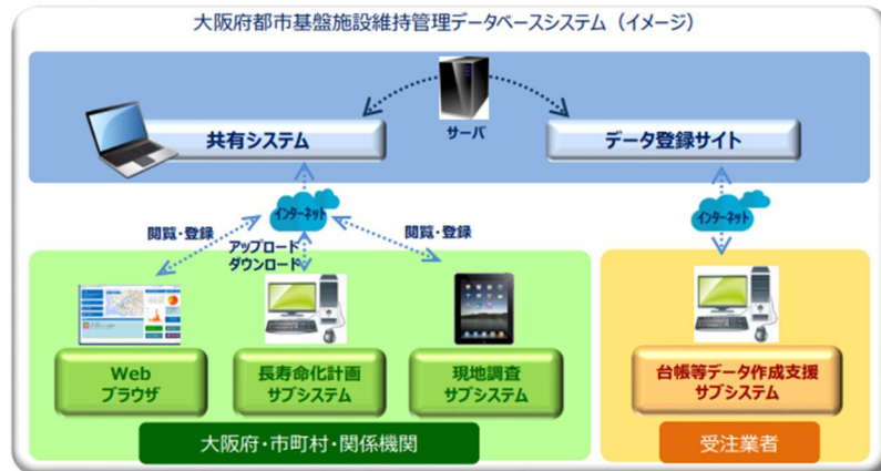
図 2.1-9 大阪府維持管理データベースシステムの概要
