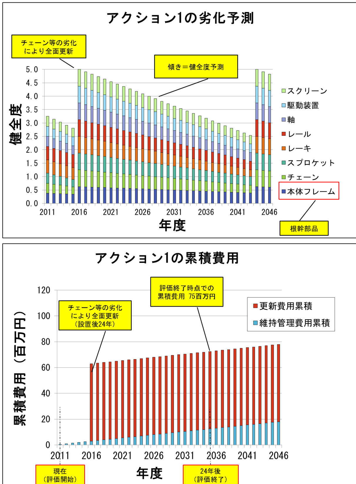
図 3.2-14 アクション1の劣化予測及び累積費用
