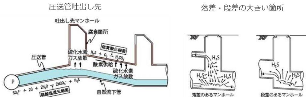
図 3.1-5 腐食の恐れのある大きい箇所
