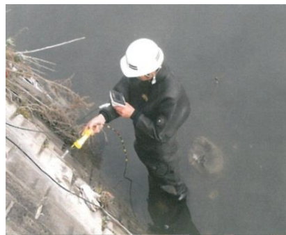
図 3.1-10 コアボーリング、カメラによる空洞化調査
