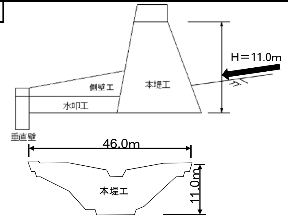
標準断面図
