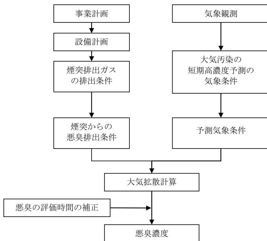
図 6-1.15 煙突排出ガスによる悪臭の予測手順
