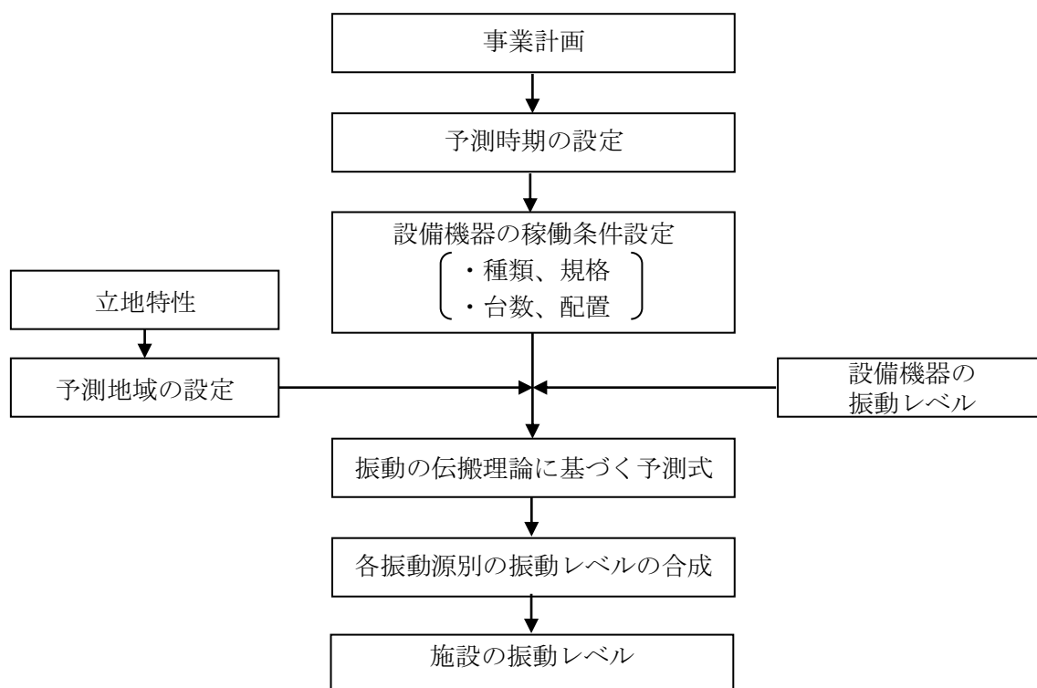
図 6-1.13 施設の稼働による振動レベルの予測手順
