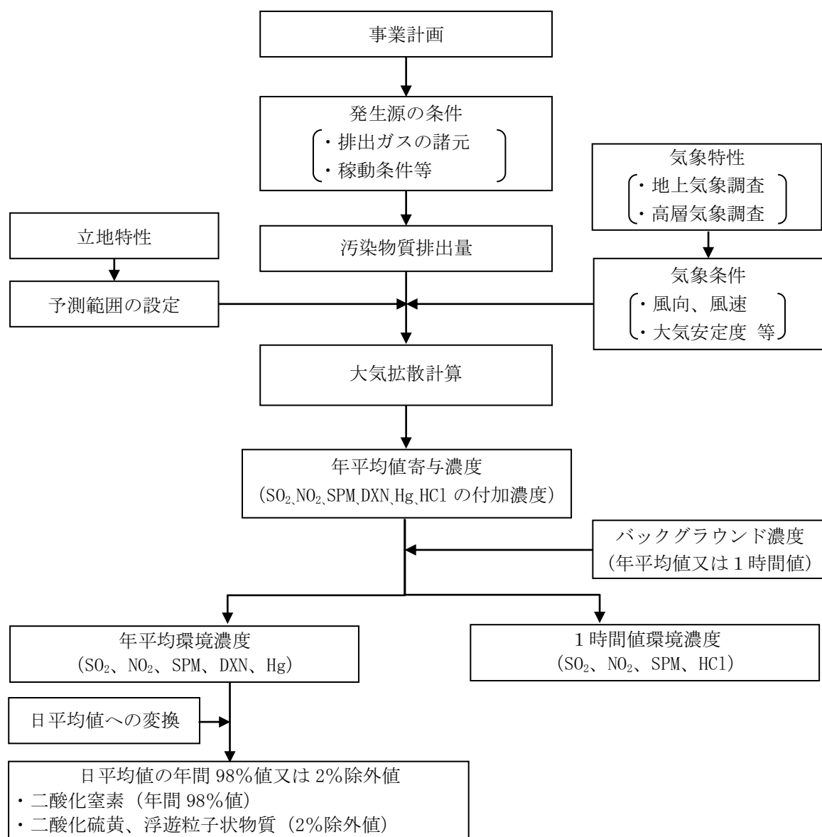
図 6-1.5 施設の稼働による大気質の予測手順
