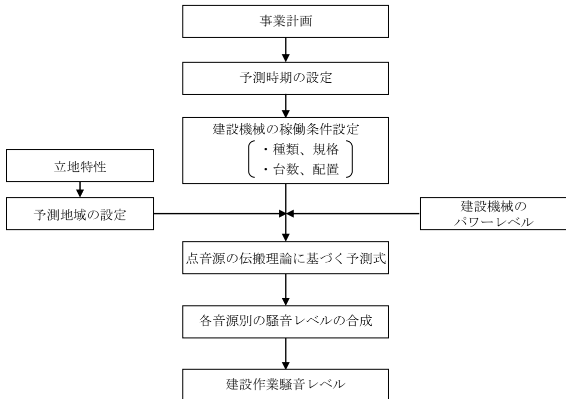
図 6-1.8 建設機械の稼働による騒音レベルの予測手順
