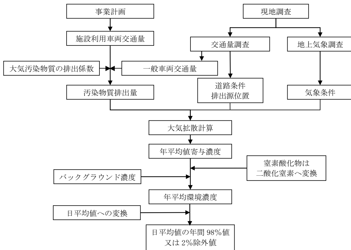
図 6-1.6 施設利用車両の運行による大気質の予測手順
