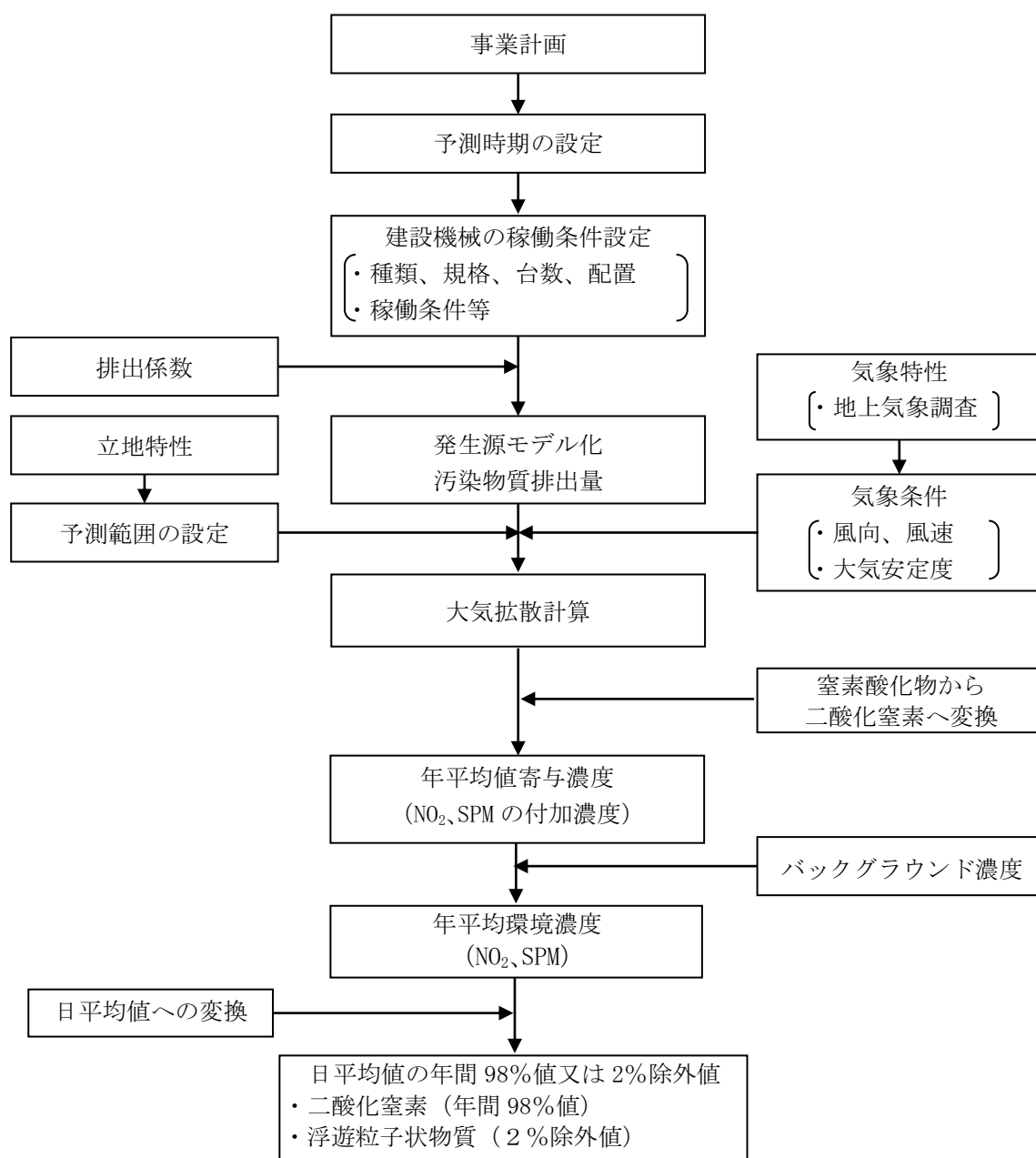
図 6-1.3 建設機械の稼働による大気質の予測手順
