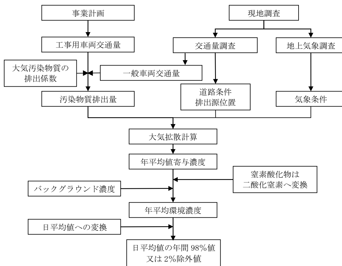
図 6-1.4 工事用車両の運行による大気質の予測手順
