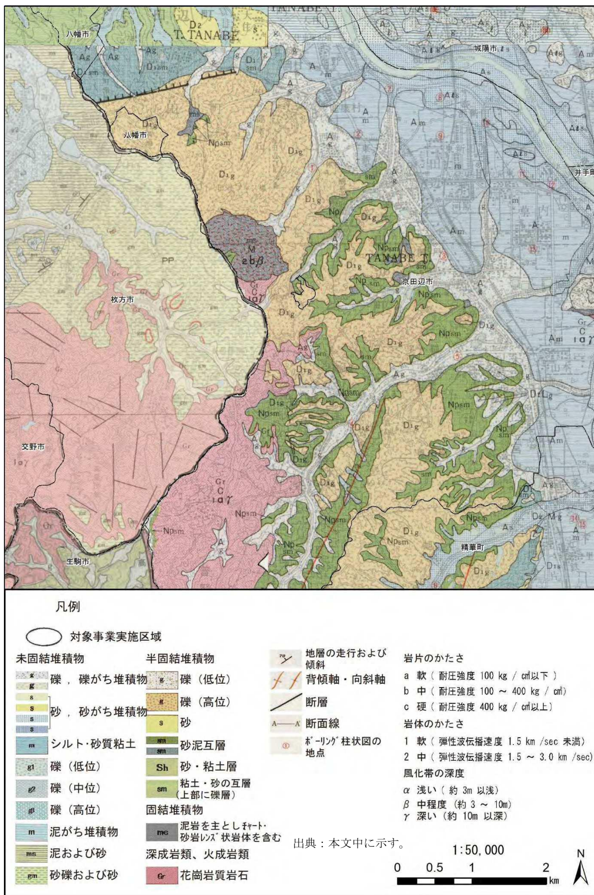
図 2-2.11 地質図
