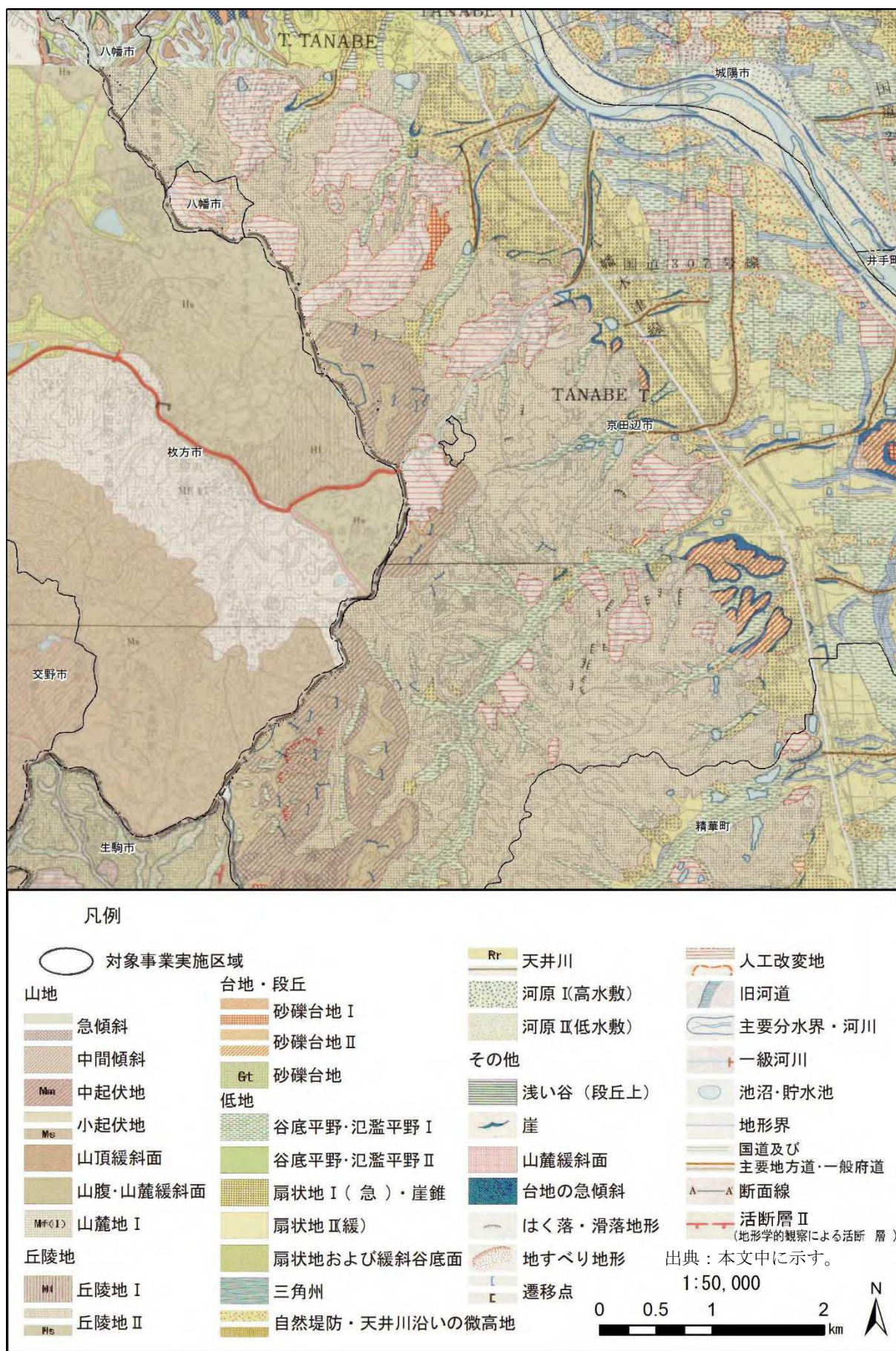
図 2-2.10 地形図
