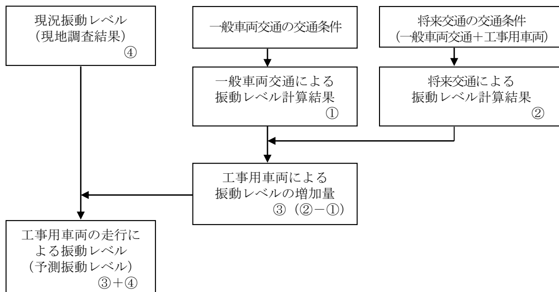
図 6-1.12 工事用車両の運行による振動レベルの予測手順
