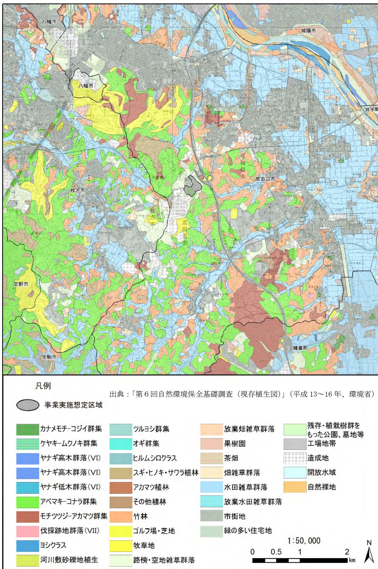
図 2-2.13 現存植生図
