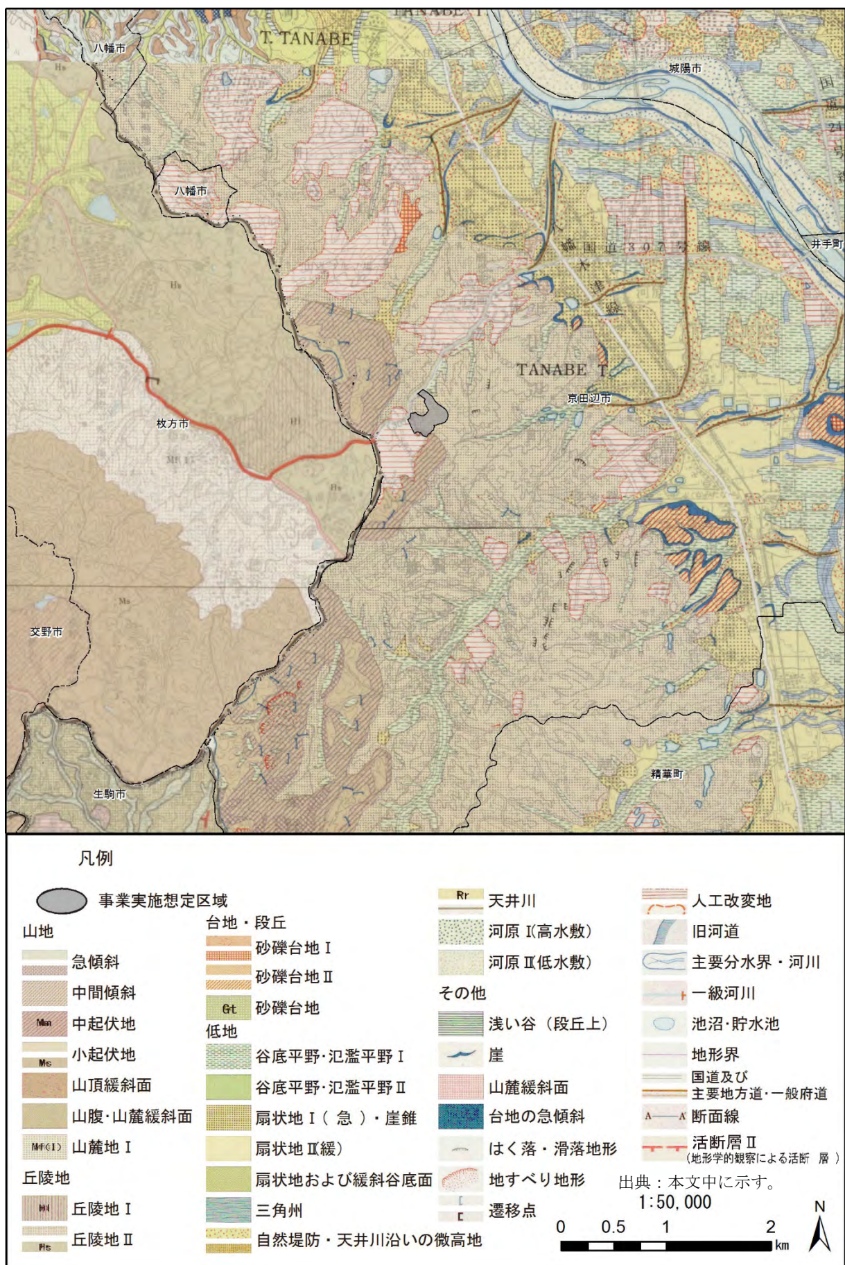
図 2-2.10 地形図
