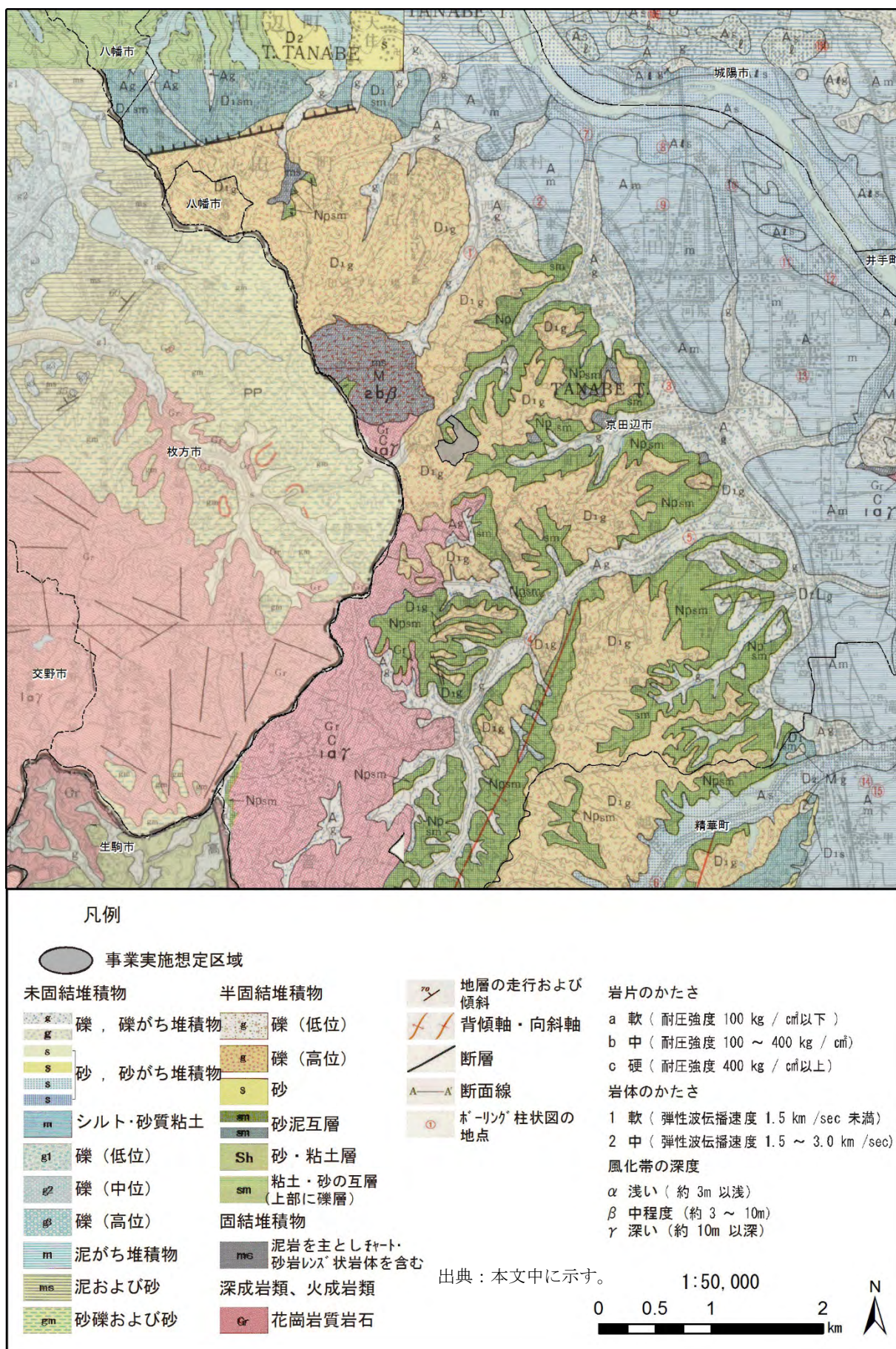
図 2-2.11 地質図
