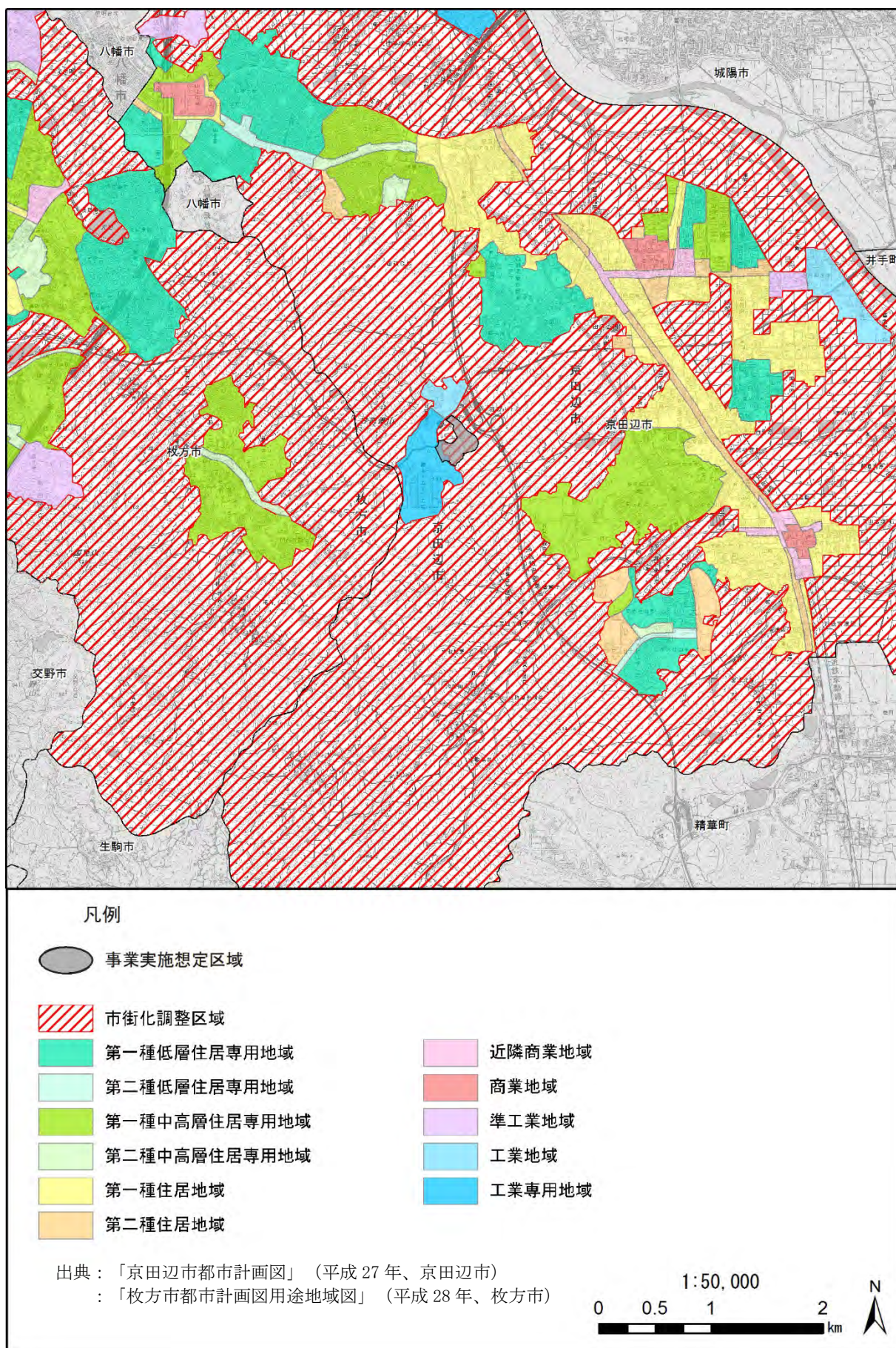
図 2-2. 26 用途地域図
