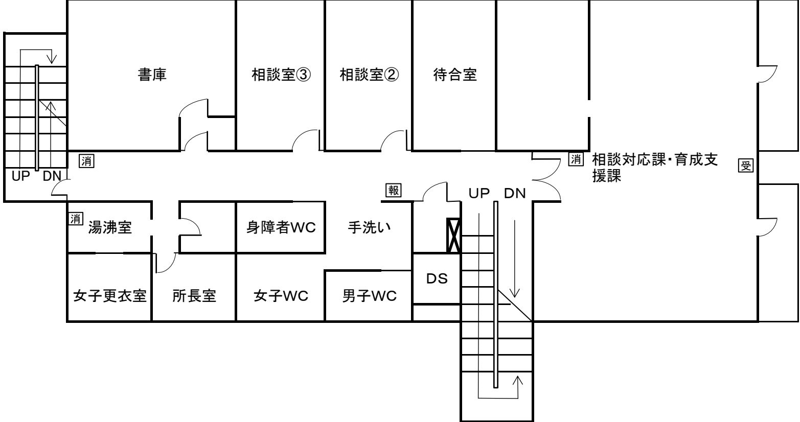
(2階平面図)
