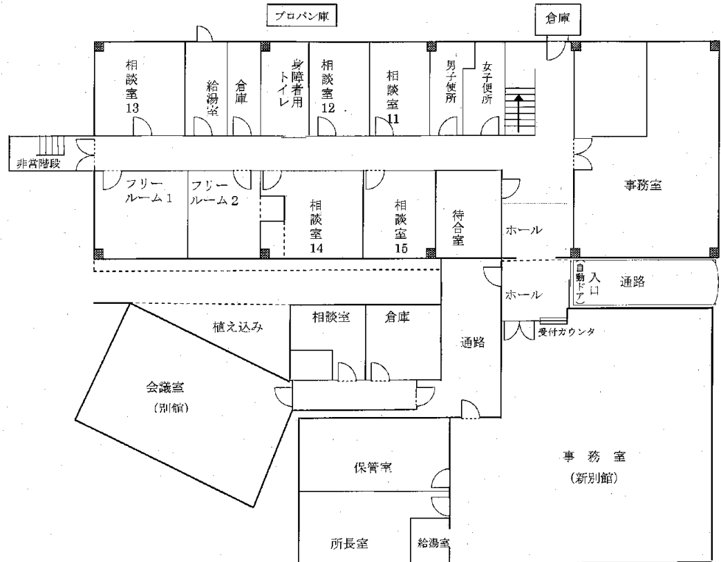
(本館 1 階平面図)
