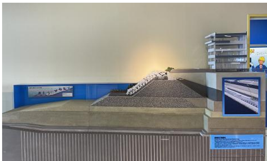
緩傾斜石積護岸の模型（写真提供：関西エアポート株式会社）
