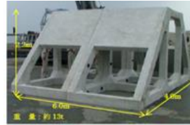
図 23 攪拌ブロック礁
