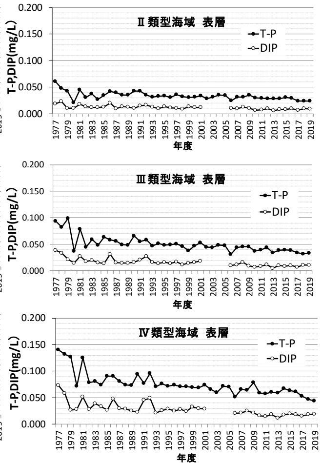
図 16 表層の全リン(T-P)及び溶存性無機態窒素(DIP)の年平均値(mg/L)の経年変化 (大阪府が測定する環境基準点におけるデータ)
