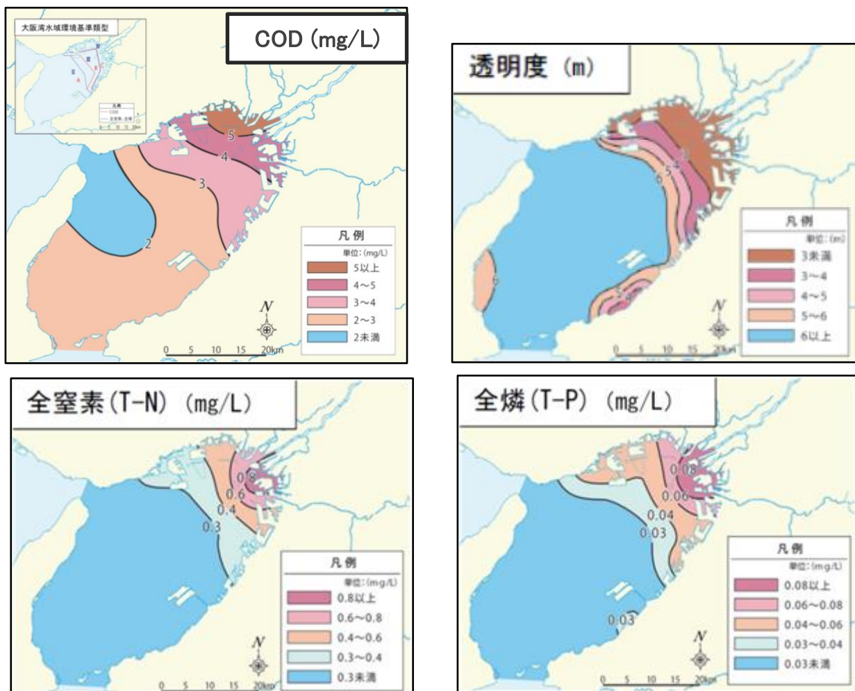
図 17-1 夏季の表層 COD 濃度、透明度、全窒素、全りん分布 （平成 28 年～30 年度、6～8 月平均）
