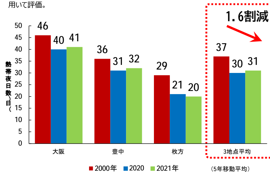
図2 地球温暖化の影響を除外した熱帯夜日数の比較 (気象庁データより大阪府作成)
