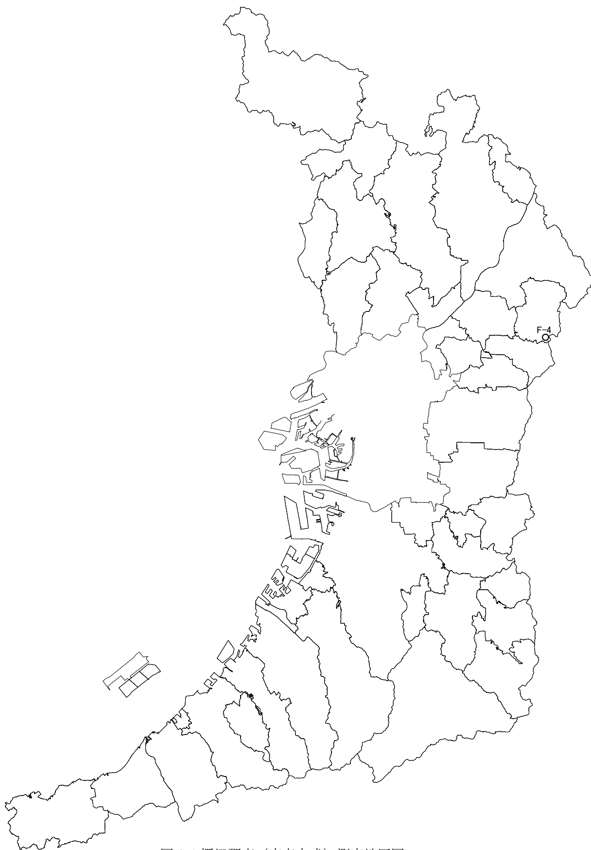
図 2-1 概況調査（定点方式）測定地区図 （平成 30 年度）
