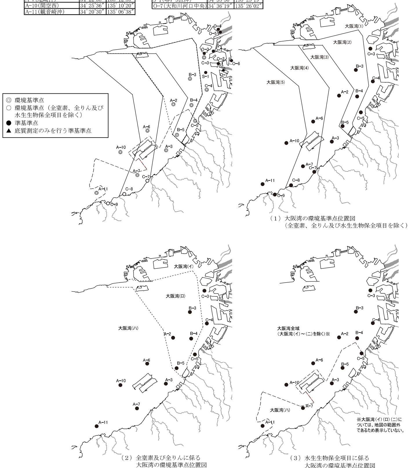
図 1 - 3 大阪湾水域の水質・底質測定地点図
