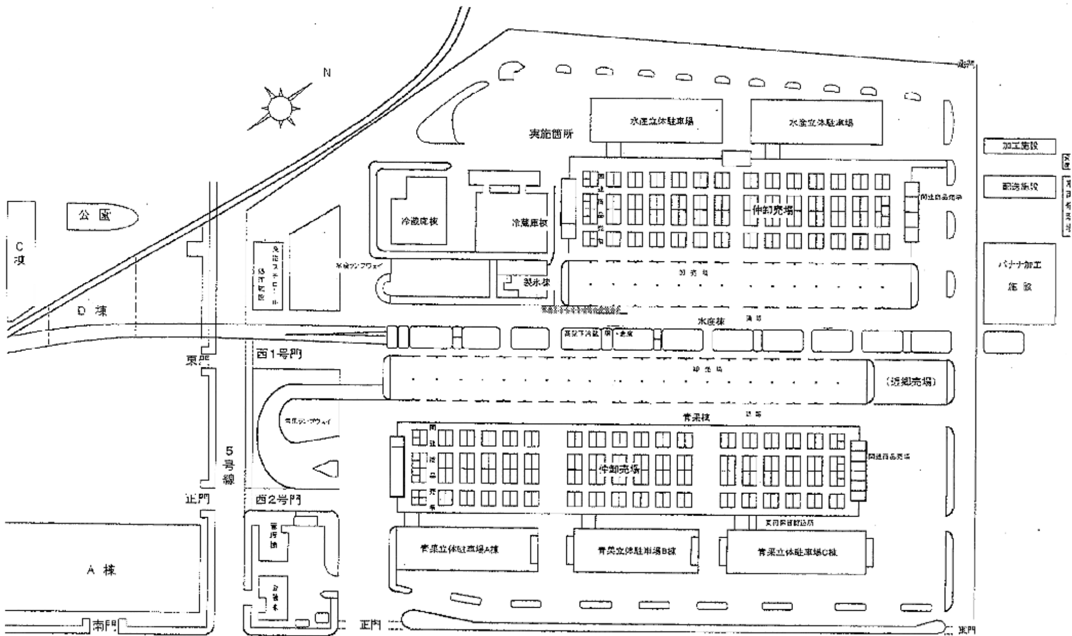
施體範書圖
