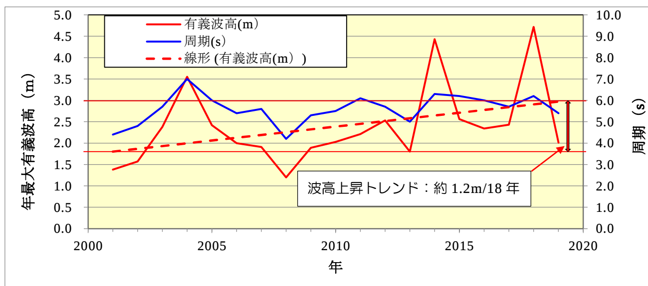
図 3-14 年最大有義波高経年変化図（神戸港：2001～2019 年）
