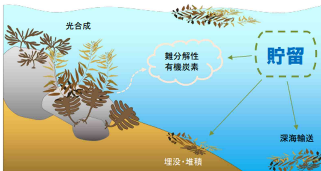
図 1-2 ブルーカーボンによる二酸化炭素吸収・貯留の仕組み（出典 水産庁HP）
