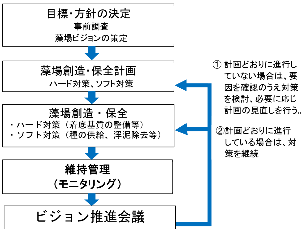
図 4-14 維持管理
