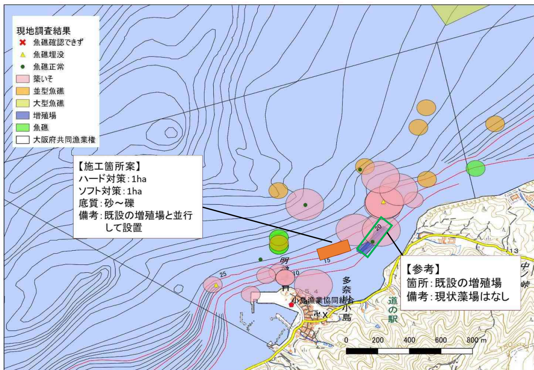
図 4-6 (11) 整備の位置図 (小島地区)
