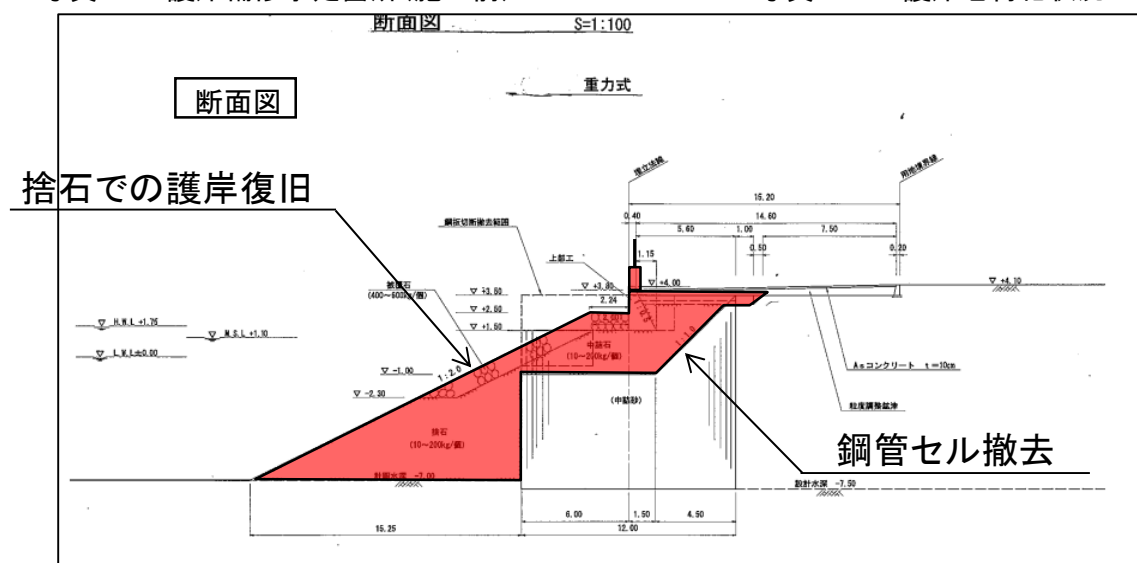
図－1 護岸補修 断面図
