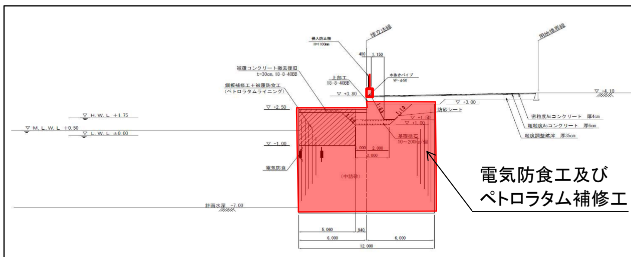
図－３ 護岸補修 断面図
