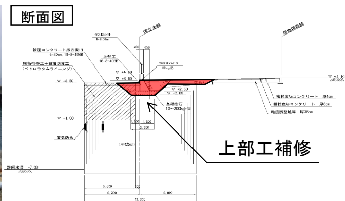
図－２ 護岸補修 断面図
