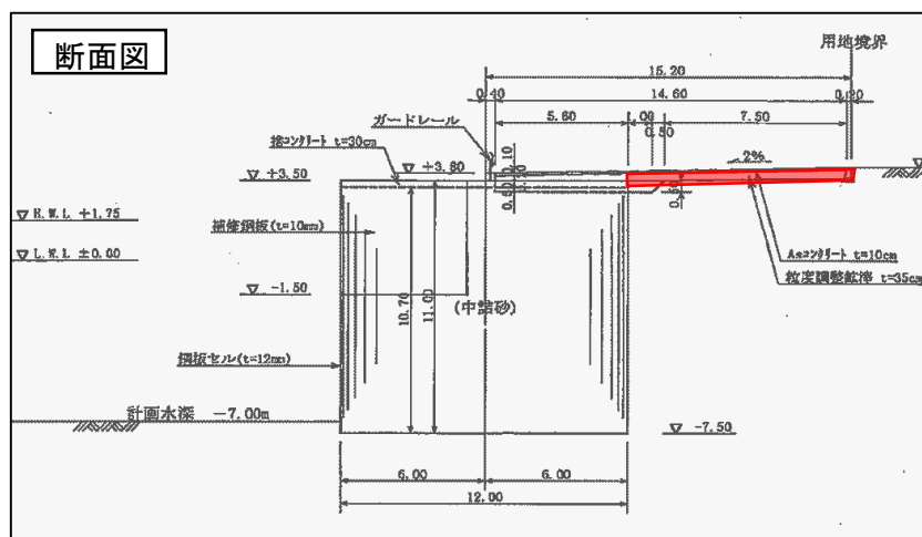
図 舗装補修 断面図
