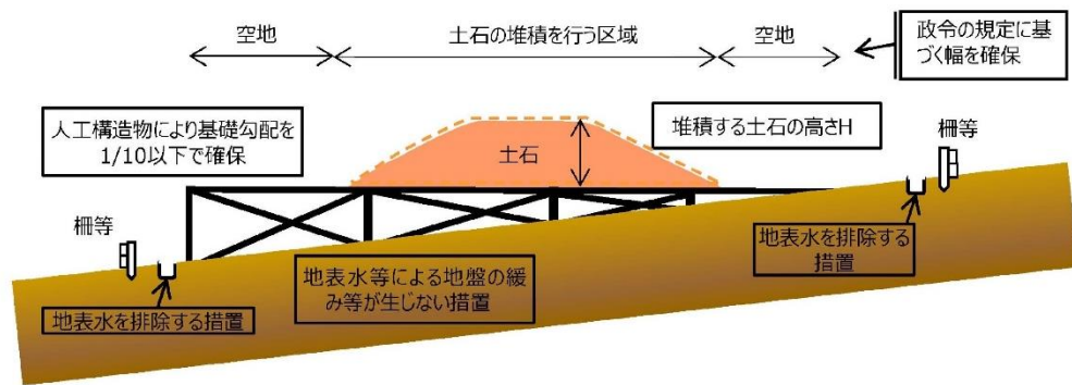
〔図－17〕 土石の堆積を行う面を有する堅固な構造物を設置する措置例
