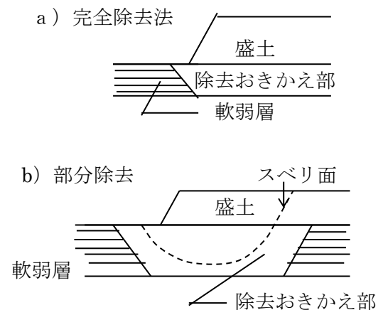
〔図－５〕 盛土の置換工法
