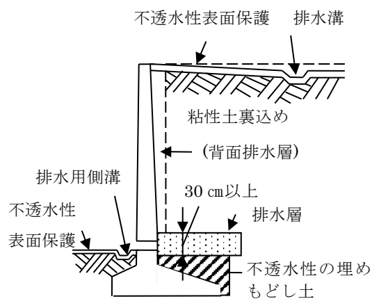
(c) 底面排水
