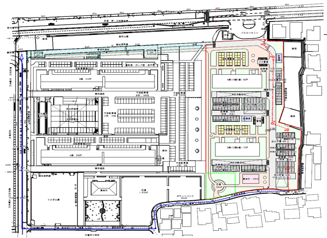
変更後建替計画図
