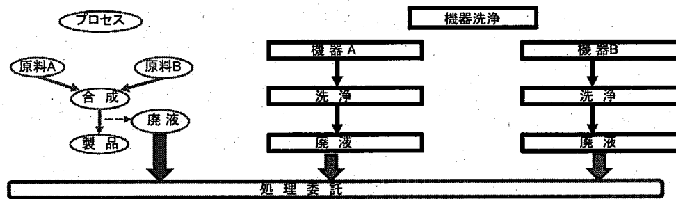
別紙(1)産業廃棄物発生工程フロー
