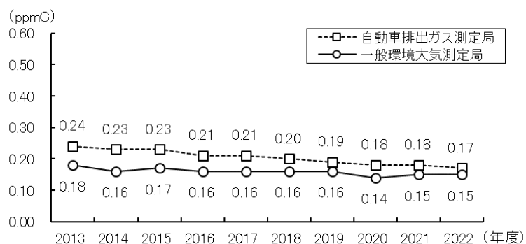
非メタン炭化水素濃度の推移 (午前6時から午前9時の3時間平均値の年平均値)
