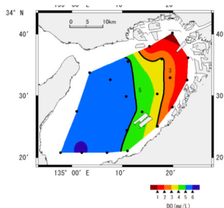
夏季底層 DO の分布図(2020~2022 年度平均) 【提供元】(地独)大阪府立環境農林水産総合研究所
