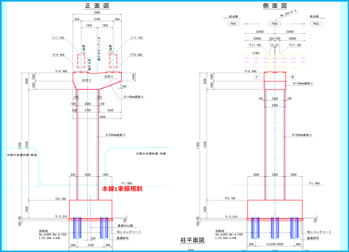
P942橋脚 構造図
