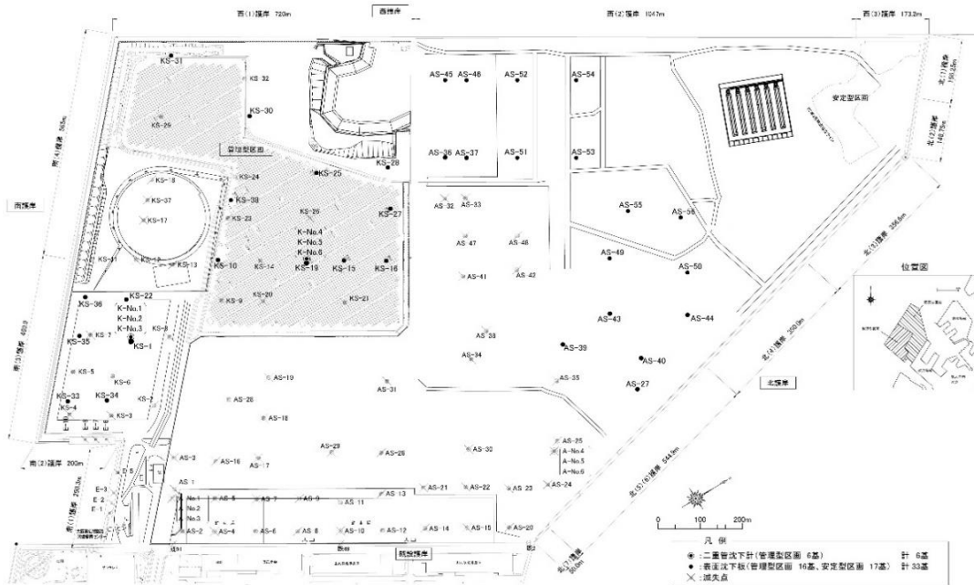
図-3.1 泉大津沖埋立処分場 表面沈下板平面位置図 (平成31年度)
