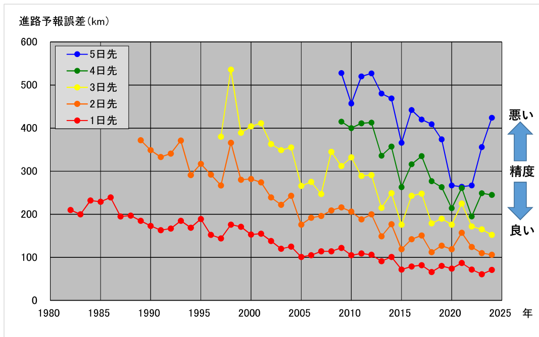
図 4 台風進路予報誤差の経年変化
