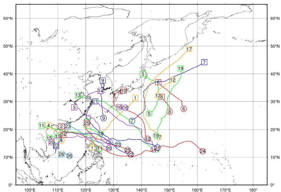
図3 2024年（令和6年）の台風経路図
