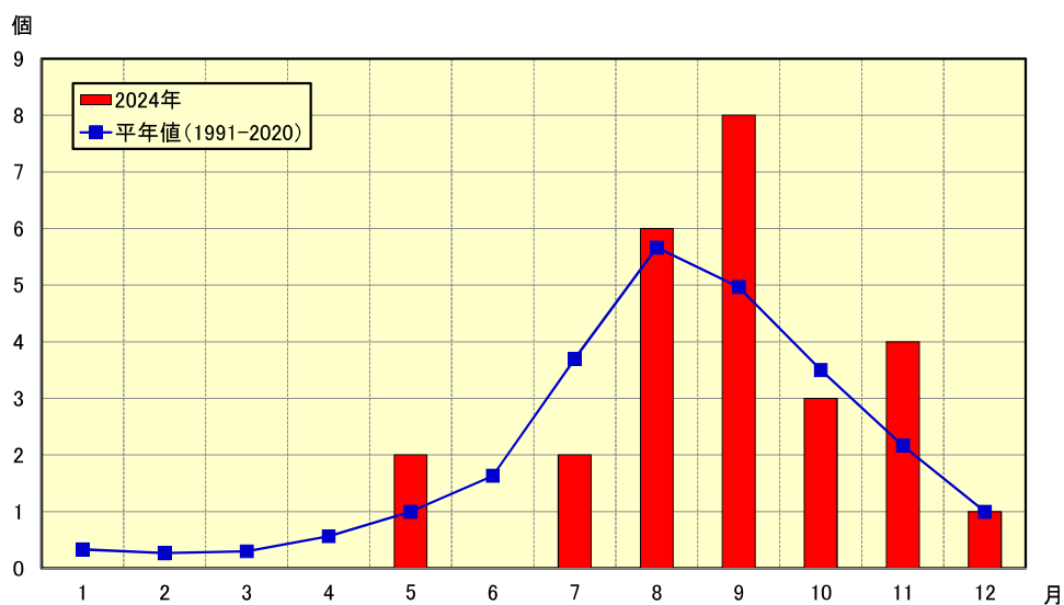
図2 2024年（令和6年）の月別発生数
