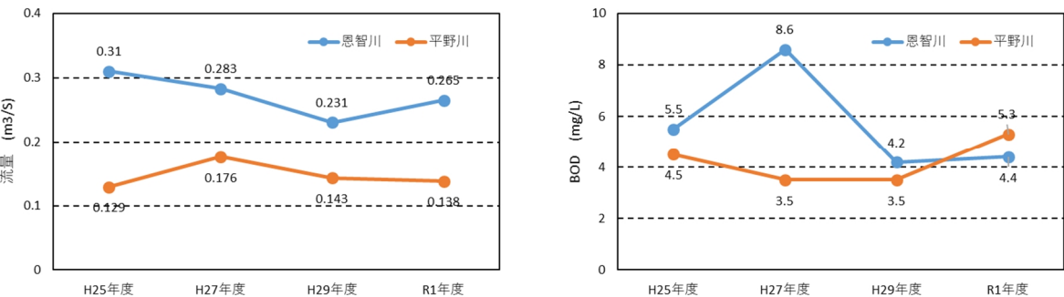
図 1.11 地下水導水地点下流の河川水量・水質(左：水量、右：水質(BOD))
