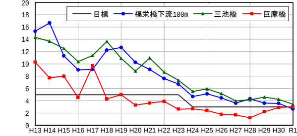
(mg/L) BOD(10~5月平均)恩智川・第二寝屋川(非感潮区間)
