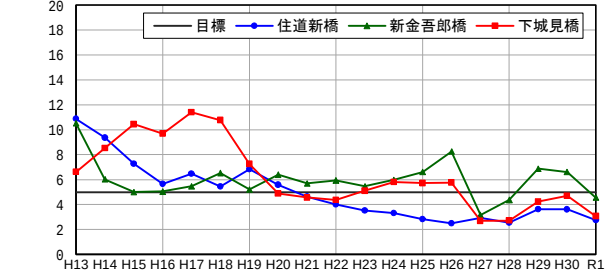
(mg/L) BOD(10~5月平均)恩智川・第二寝屋川(感潮区間)
