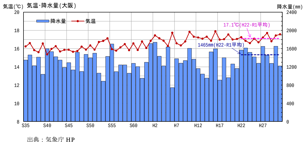
図 2.2 降水量・気温の経年変化(気象台大阪観測所)
