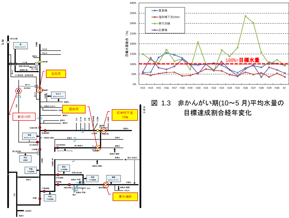
図 1.4 直近3カ年 水量目標未達成地点
