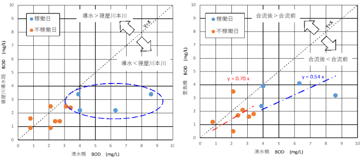
図 1.7 清水橋と浄化導水路、清水橋と萱島橋の BOD の関係
