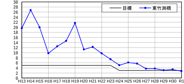
(mg/L) BOD(10~5月平均)恩智川・第二寝屋川(非感潮区間)
