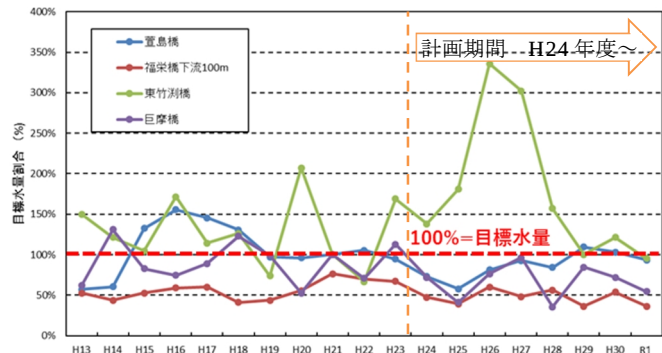
図 2.19 各地点の水量目標の達成状況 (実績水量と目標水量の比率)
