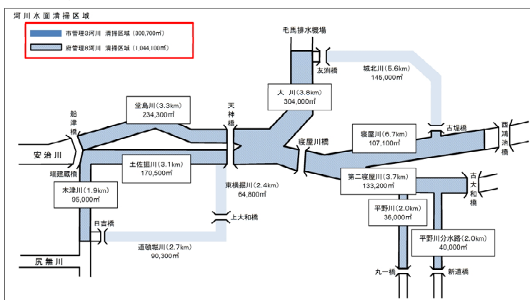
図 5.16 大阪府、大阪市による浮遊ごみの回収範囲 (寝屋川流域外を含む)
