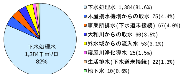
図 2.14 寝屋川流域の流入水の内訳
