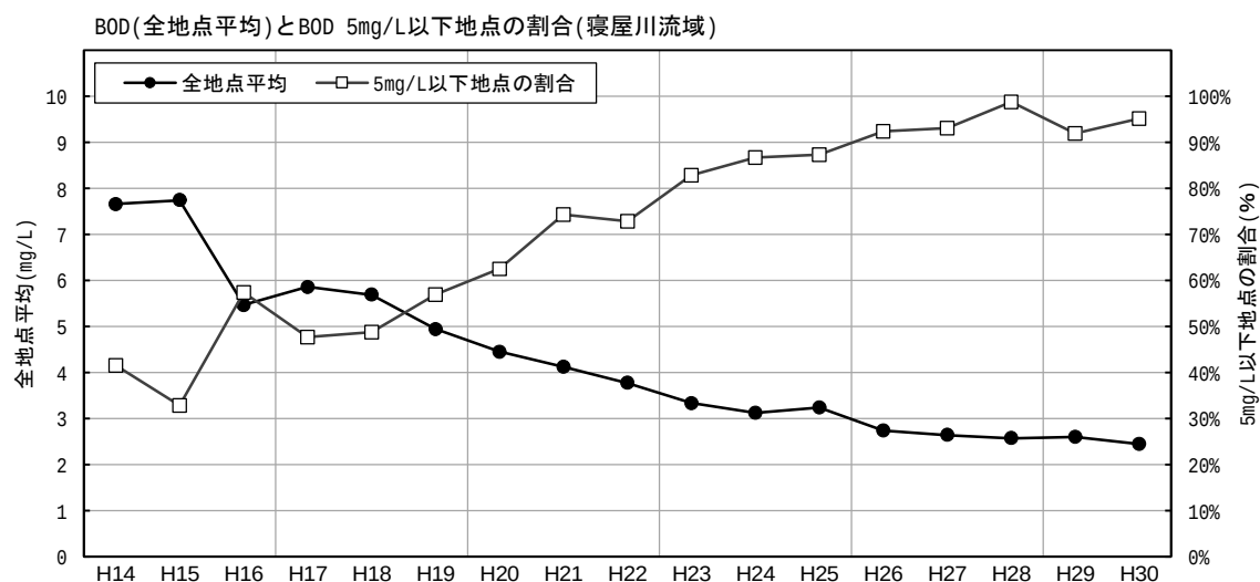
図 2.9 全地点平均水質(BOD 年平均値)と BOD 5mg/L 以下地点の割合(水質常時監視地点以外)
