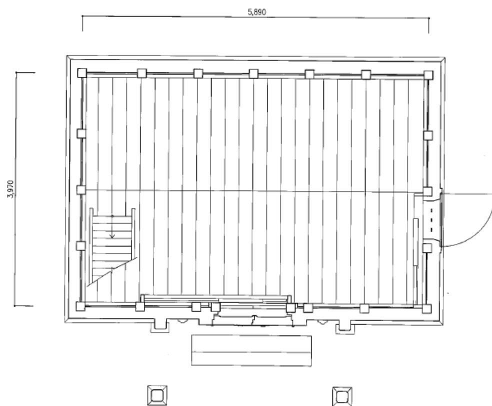
図6 御文庫平面図1階
