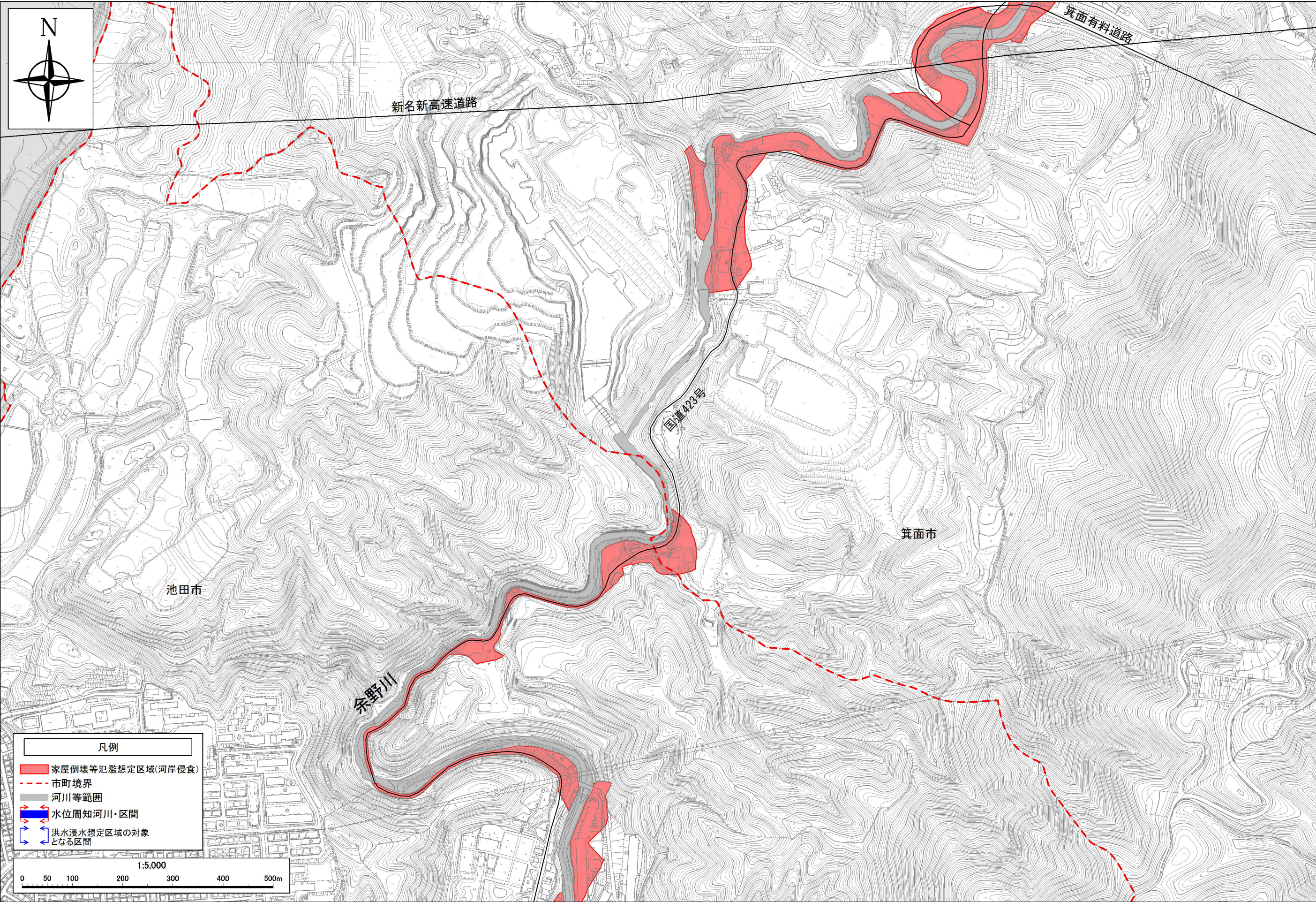
淀川水系 余野川・石田川・切畑川・木代川 洪水浸水想定区域図(家屋倒壊等氾濫想定区域(河岸侵食)) 拡大図3
