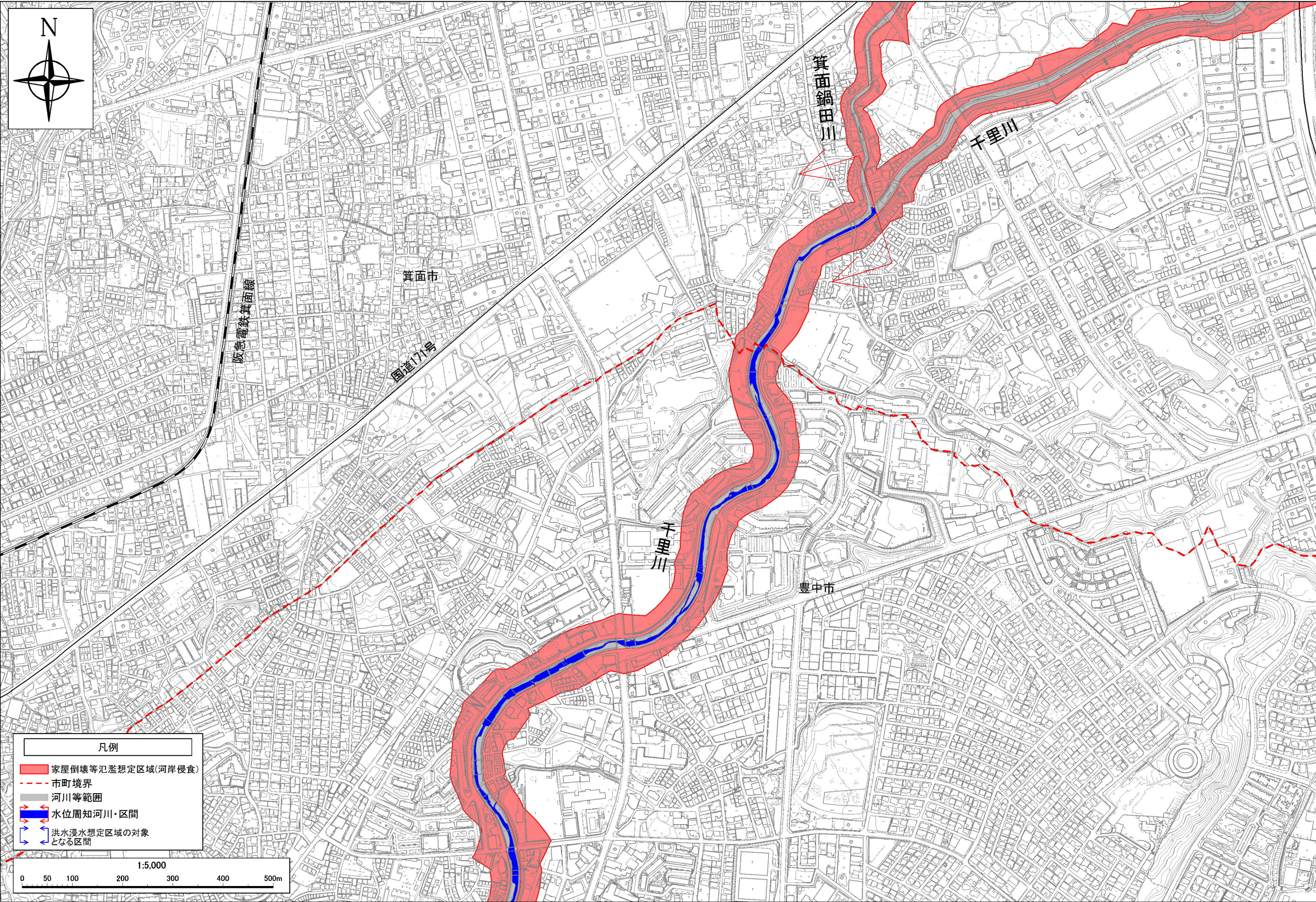
淀川水系 千里川・芋川・箕面鍋田川 洪水浸水想定区域図(家屋倒壊等氾濫想定区域(河岸侵食)) 拡大図4
