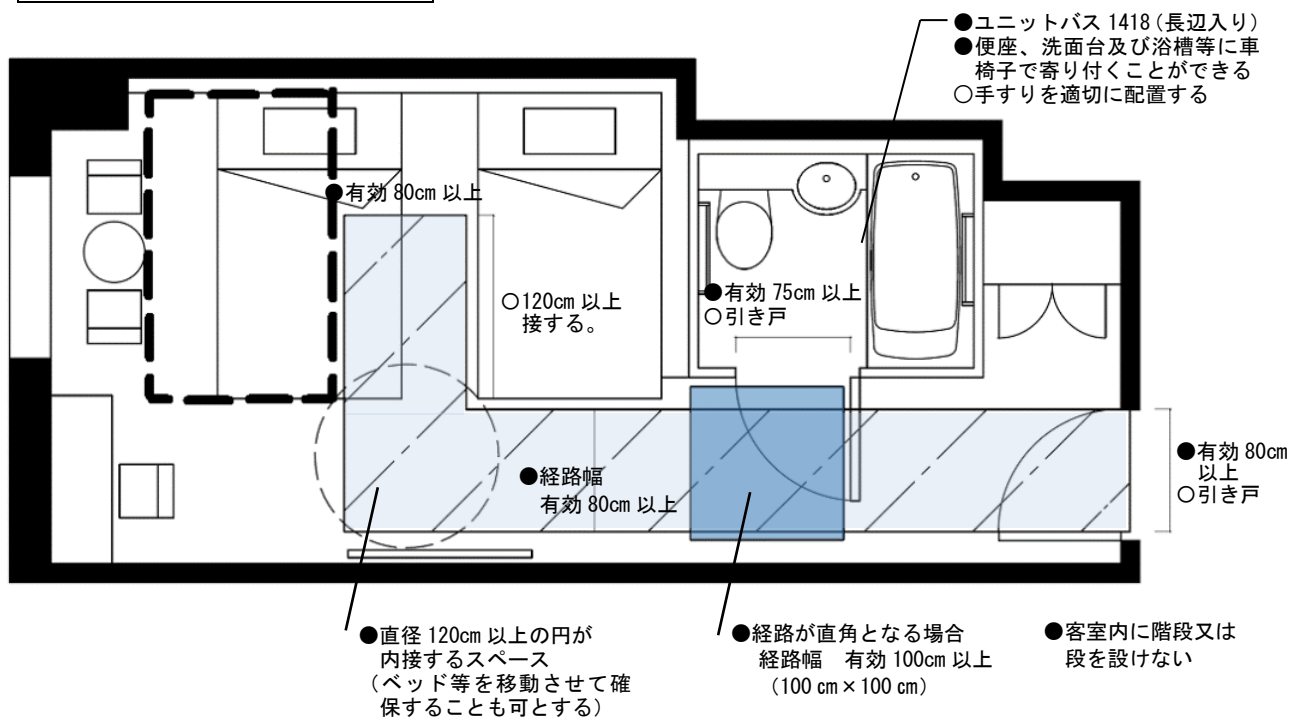
UD ルームⅡ（客室面積 22.2 m 2 ）
