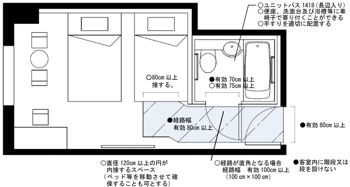
UD ルームⅡ（客室面積 22.2 m 2 ）
