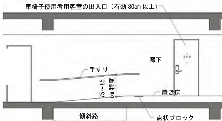
廊下縦断面
