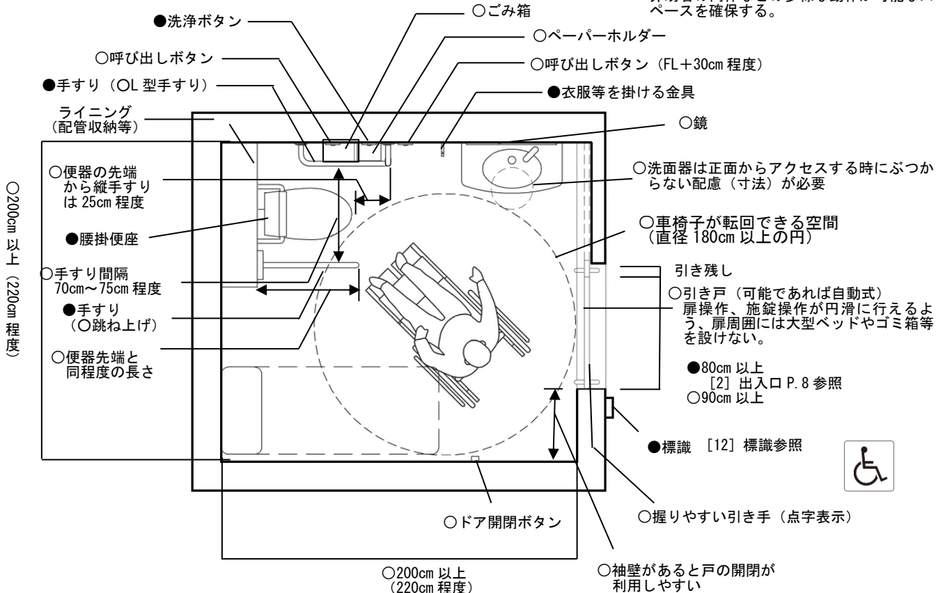
○2,000 m 2 以上の特別特定建築物の車いす使用者用便房の計画例
