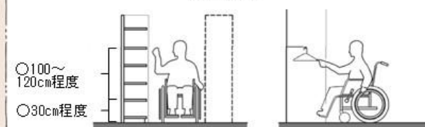
（通路断面）
