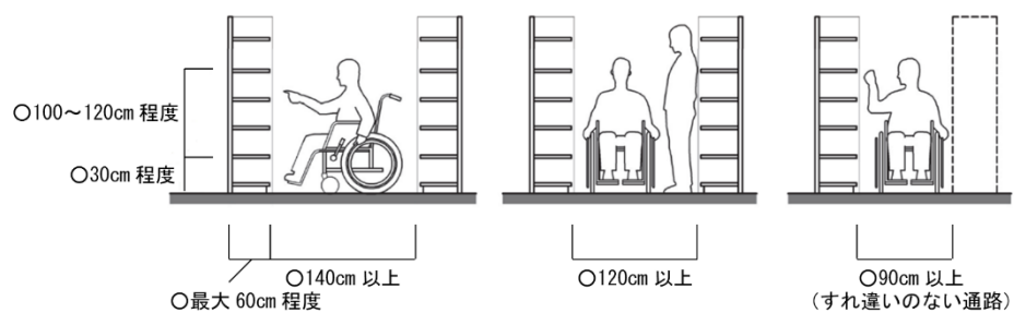
物販店舗の通路の例
