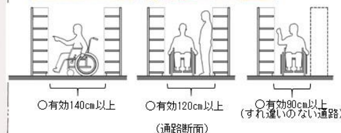
（通路断面）
