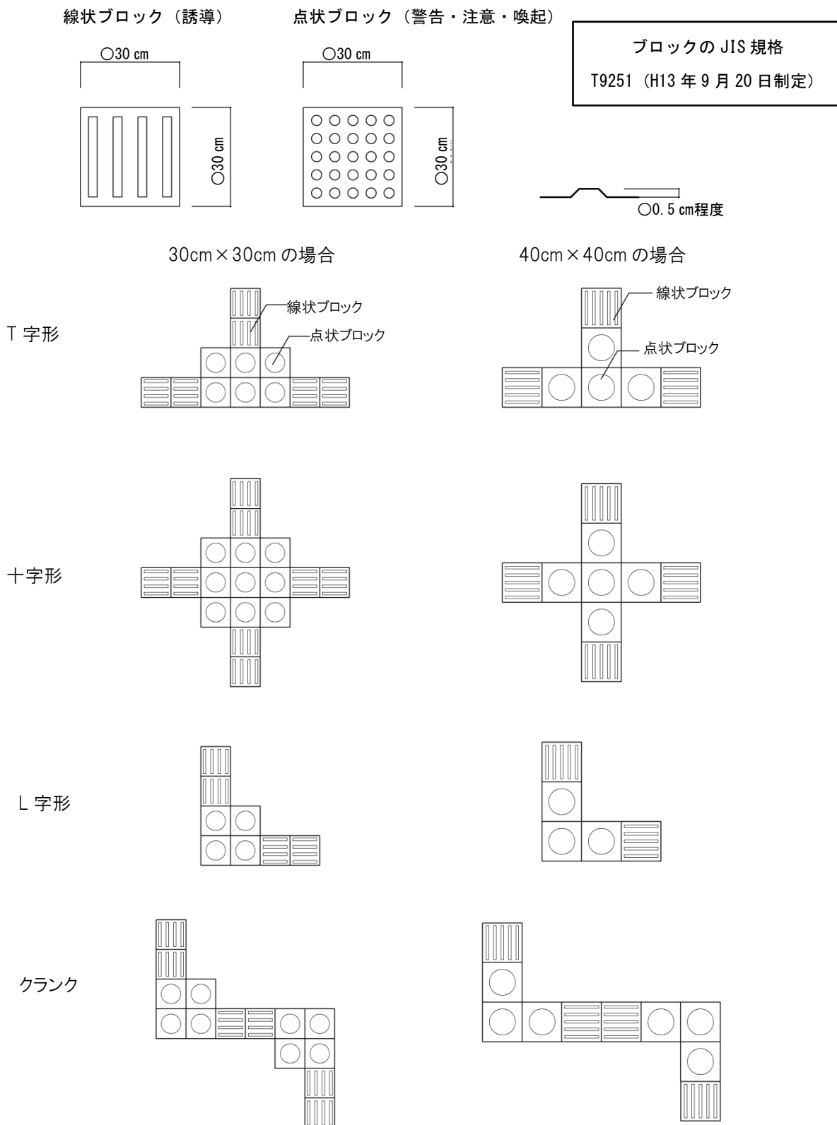
○図 14.6 視覚障がい者誘導用ブロック等
