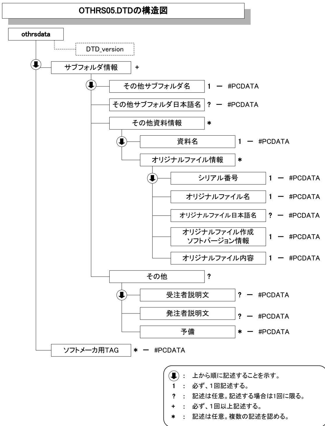
図付 1-3 その他管理ファイルの DTD の構造
