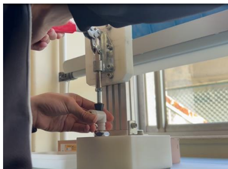
機械の導入により、組立作業が効率的に
