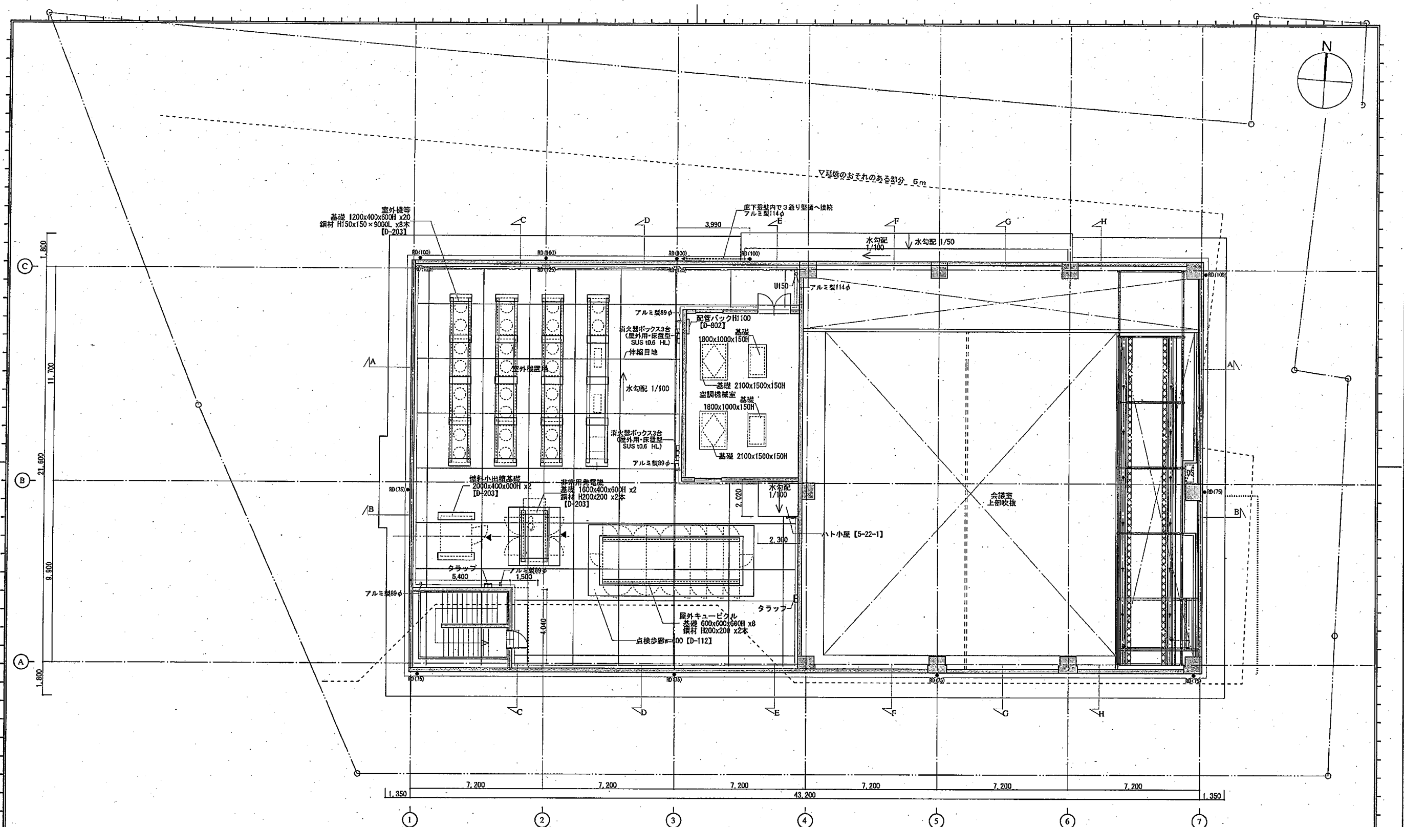
塔屋階平面図
