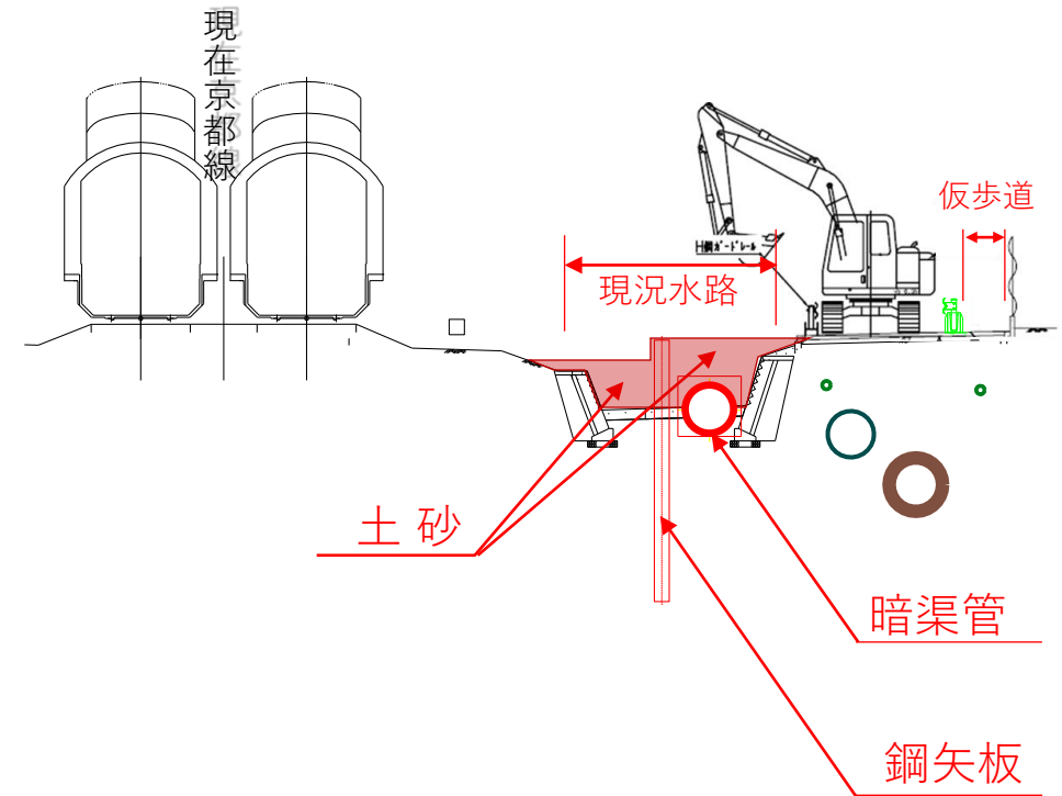
水路横断図
