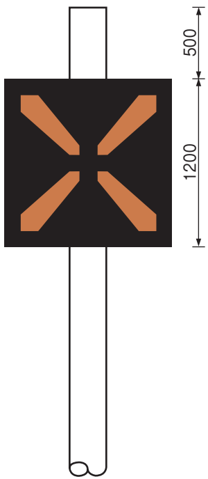
【信号柱の標識】
