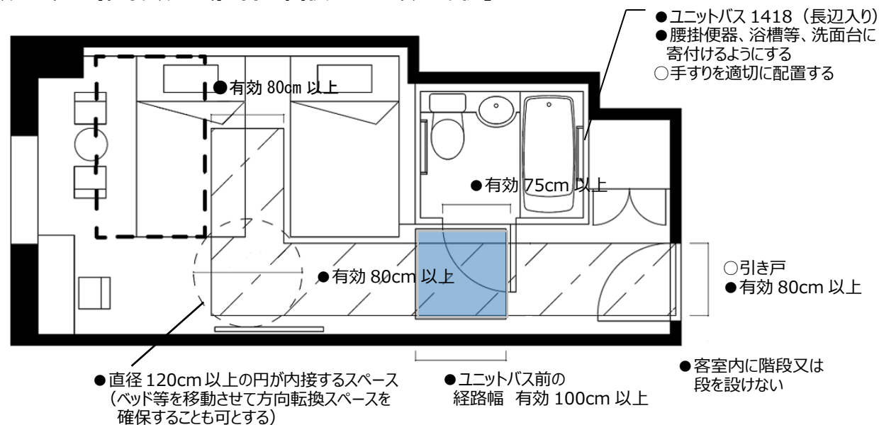
【UD ルーム II（ツインルーム）客室面積 22 m 2 以上の例】
