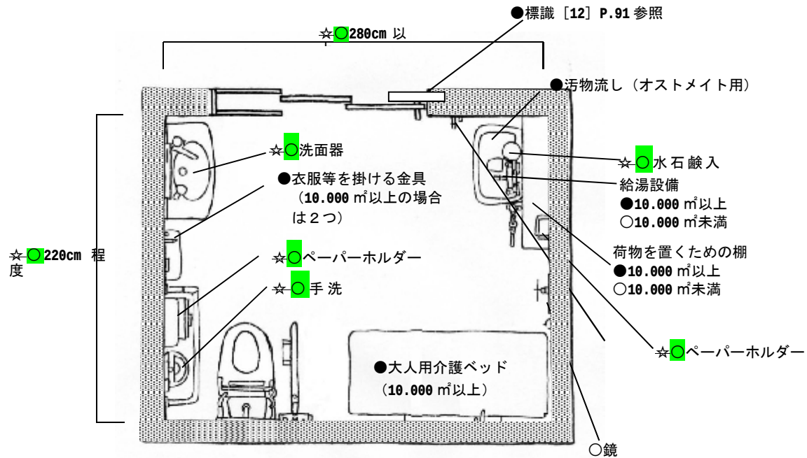
●○☆図 8.23 汚物流し（オストメイト用）及び大人用介護ベッドを 車いす椅子使用者用便房内に設けた例（220cm×280cm タイプ）
