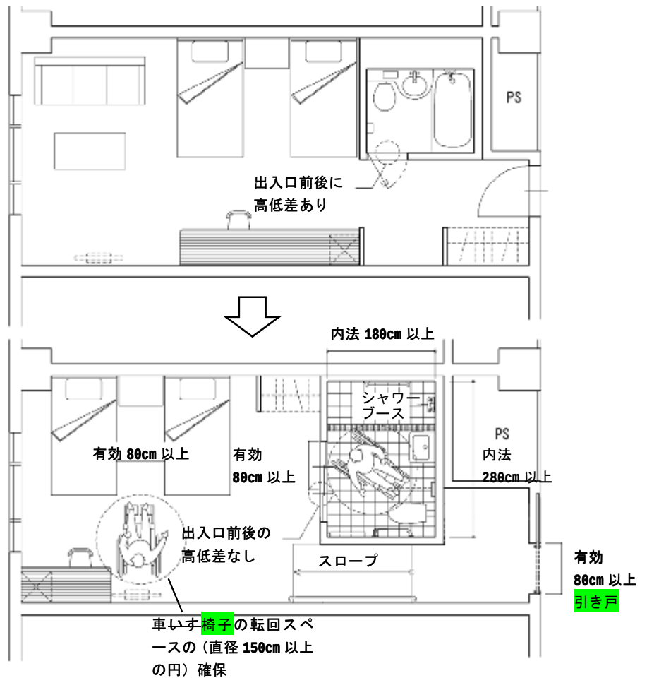
☆○図 10.1115 改善例 1（一般客室 1 室を車いす椅子使用者用客室 1 室に改善する例）
