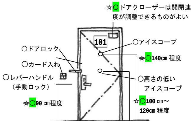
○☆図 10.5.12 客室ドアの例 (車椅子使用者用客室・一般客室)
