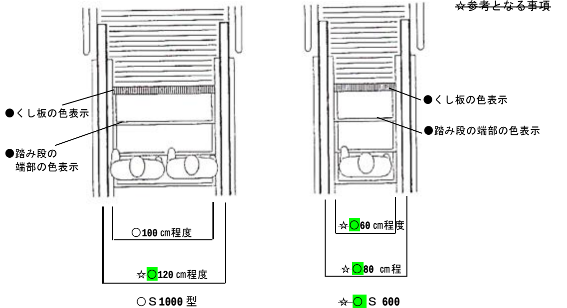
☆〇図 7.3 車いす椅子用エスカレーターの例
