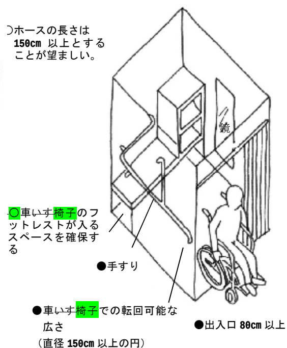
●図 11.6 更衣ブース
