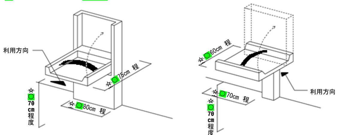
☆〇図 8.18 乳幼児用ベビーベッド
