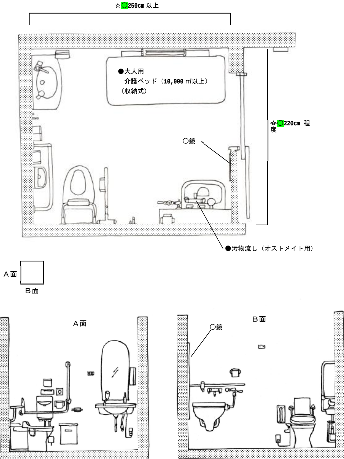
●○☆図 8.24 汚物流し（オストメイト用）及び大人用介護ベッドを 車いす椅子使用者用便房内に設けた例（220cm×250cm タイプ）
