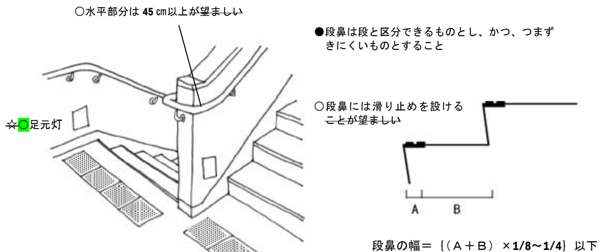
●★図 4.6 滑り止め・点状ブロック等
