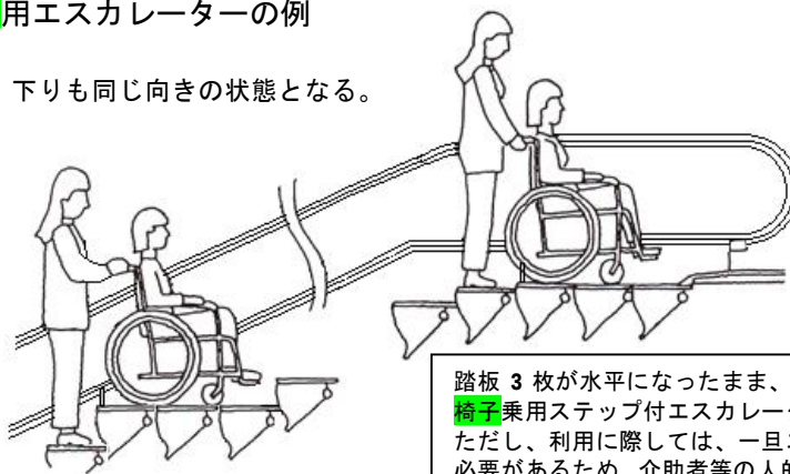
☆〇図 7.3 車いす椅子用エスカレーターの例
