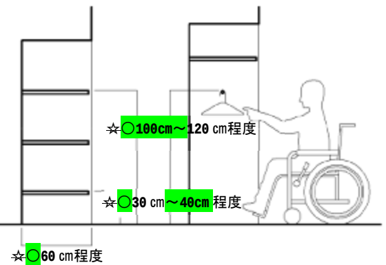
☆○図 10.8.11 収納等の高さ (車椅子使用者用客室)
