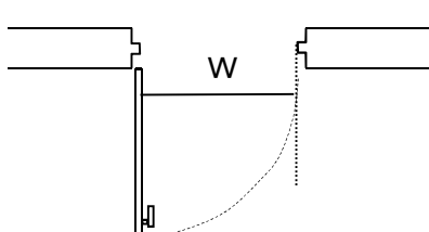
片開き戸
