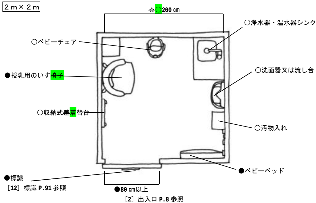
●○☆図 15.5 授乳室ベビーケアルームの例
