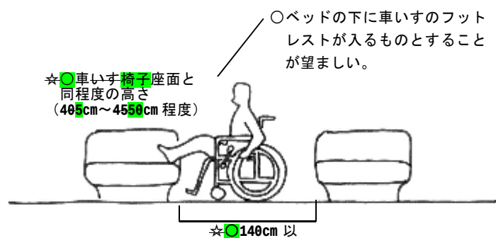
☆○図 10.6.13 ベッドの高さ (車椅子使用者用客室・一般客室)
