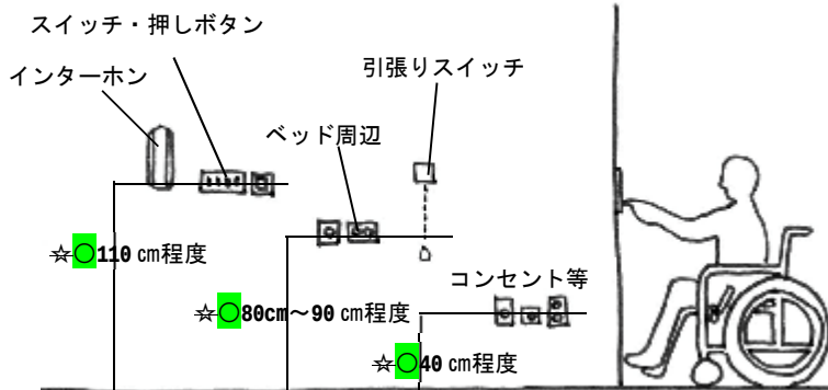
☆○図 10.7.10 コンセント、スイッチの高さ (車椅子使用者用客室)
