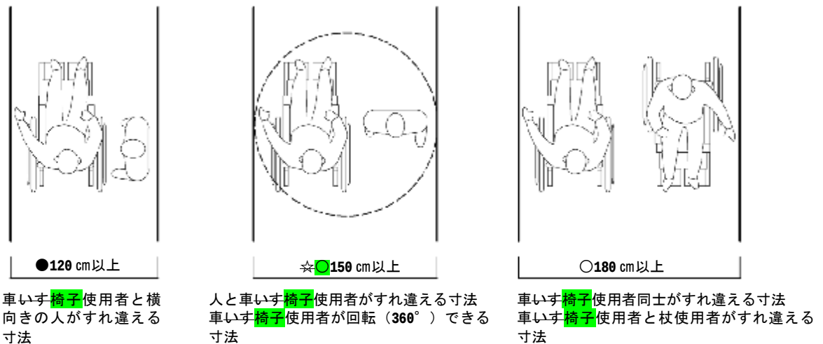
●○☆図 1.1 敷地内の通路の有効幅員
