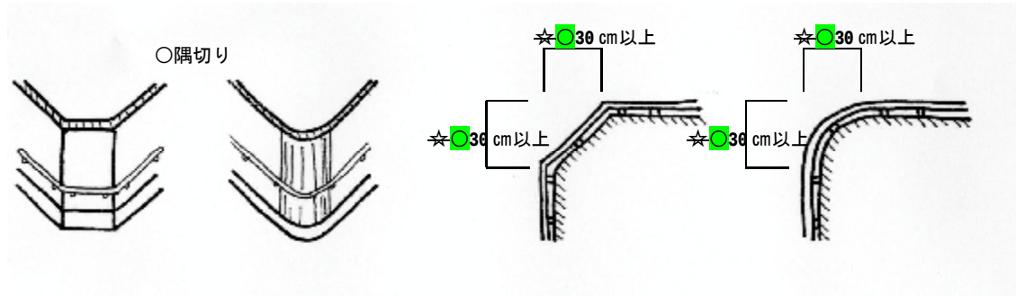
○☆図 3.6 側壁・曲がり角の隅切り
