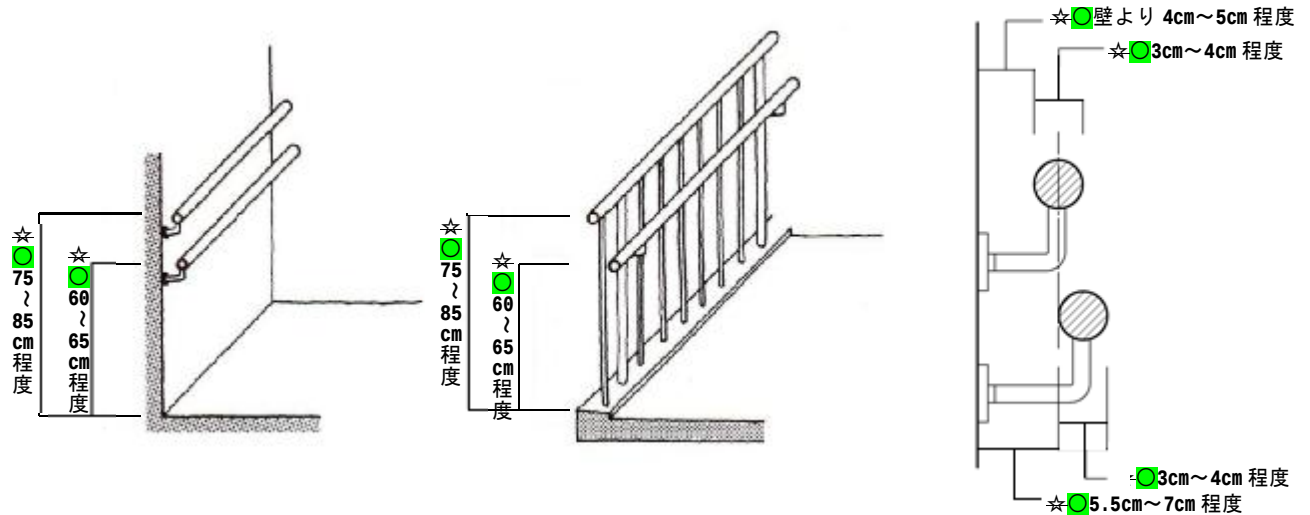
☆ 〇 図 16.1 手すりの設置寸法
