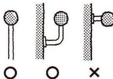
☆ 〇 図 16.2 手すりの形状
