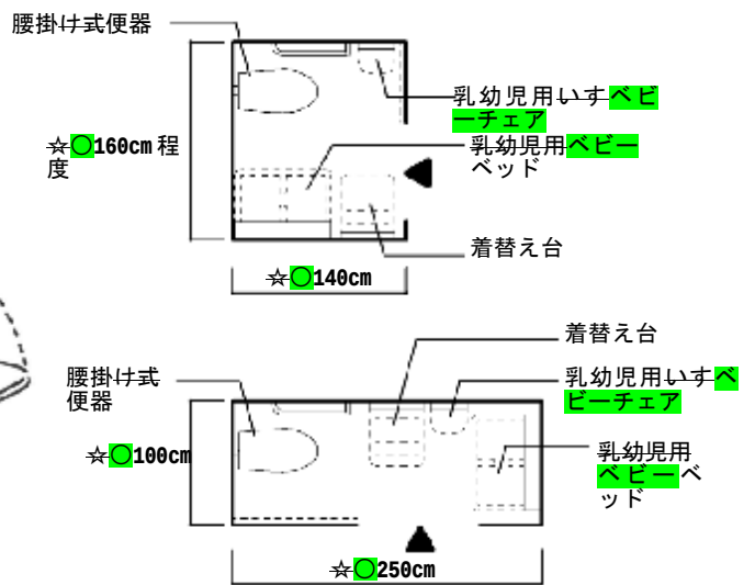
☆ 〇 図 15.4 乳幼児連れに配慮した便所の寸法例
