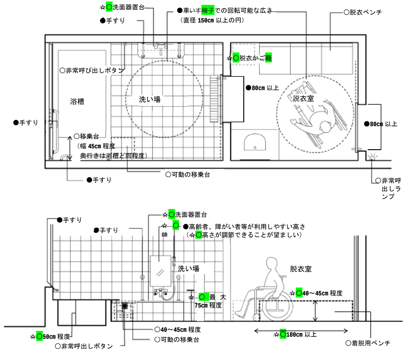
●○☆図 11.2 車いす椅子使用者が利用できる浴室の例（貸し切り浴室）
