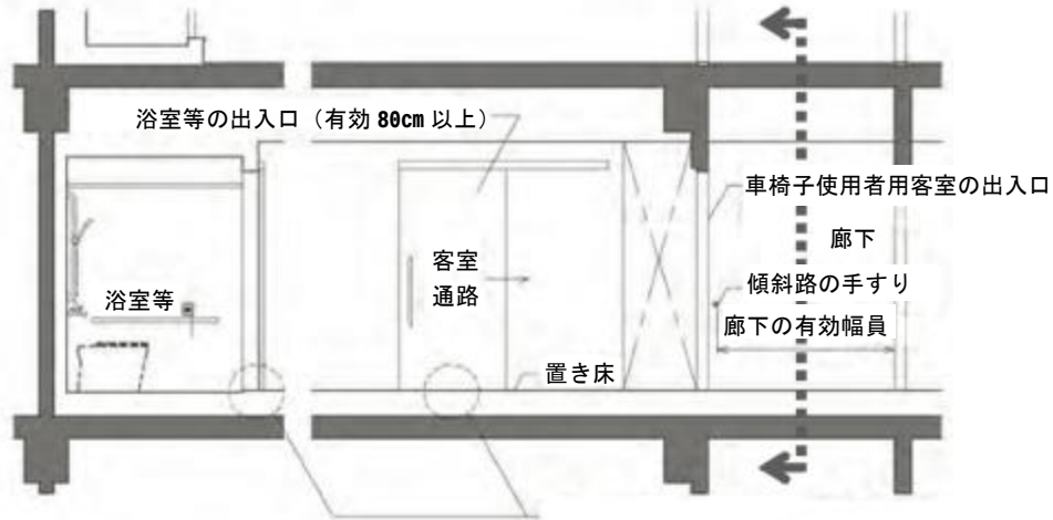
廊下縦断面
