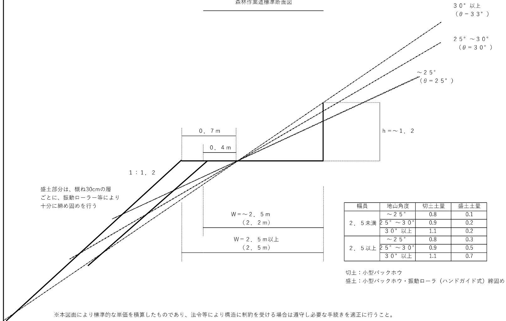
森林作業道標準断面図
